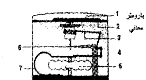
1-مقياس 2-عزل زجاجي 3-نابض 4-ميكانيكية 5-مكبس 6-غرفة 7-فراغ
