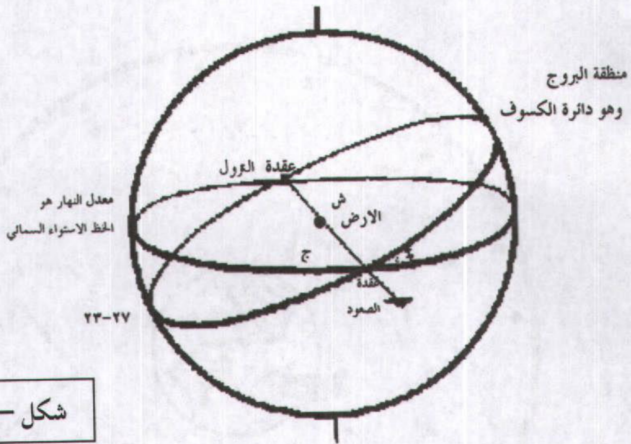
خط الاستواء السماوي ودائرة الكسوف والخسوف وموقع الارض من القبة السماوية
