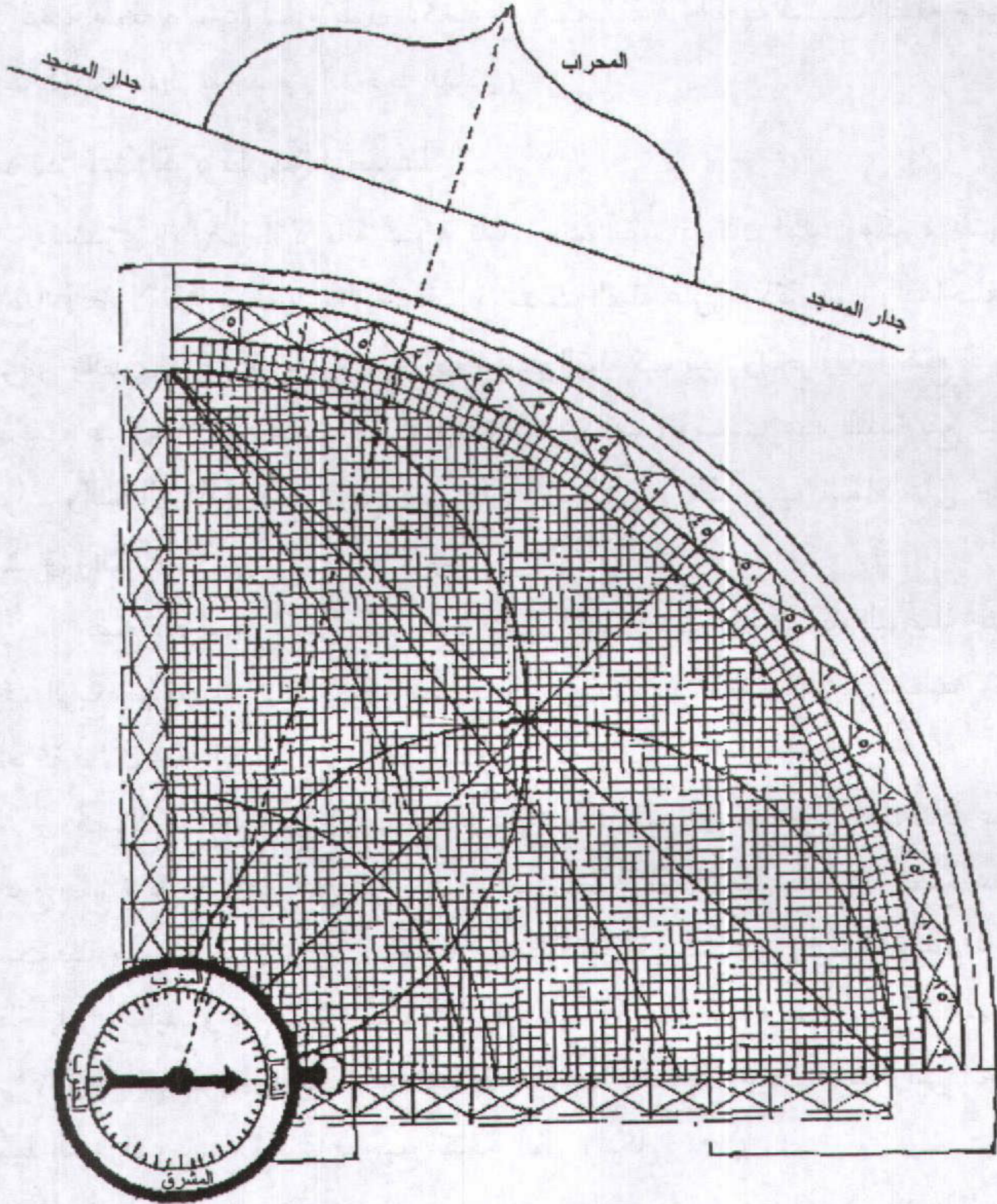
شكل - ٧٠ - لبلدة مدراس-المهند (عرضه ١٣-٠٤ درجة الشمالي وطوله ١٥-٨٠ درجة الشرقي) وسمت القبلة ١٧-٥٢ درجة الغربي الشمالي
