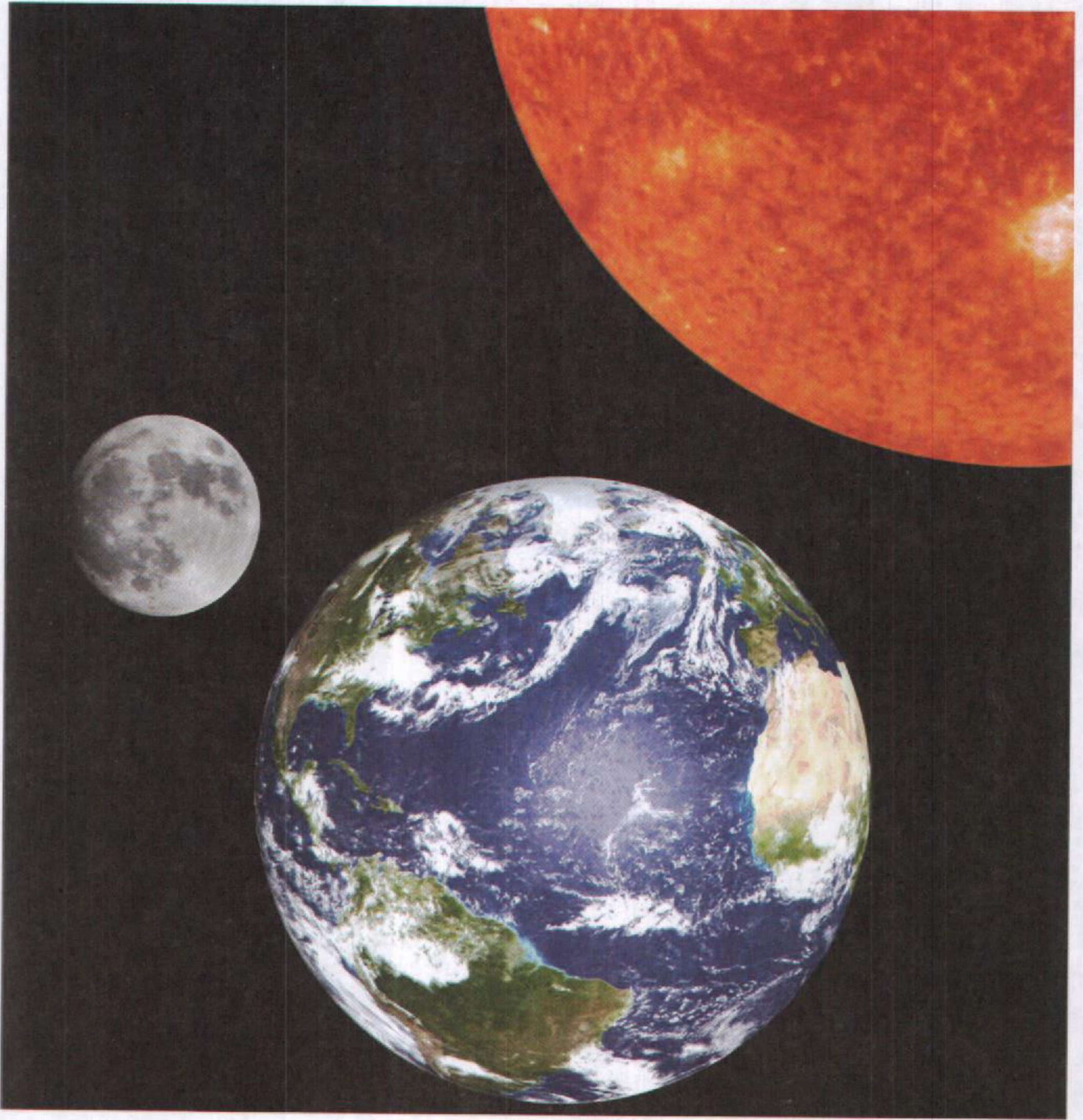
شكل - ٤١ الشمس والأرض والقمر
