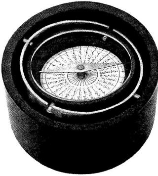
بوصلة "ابن ماجد"
