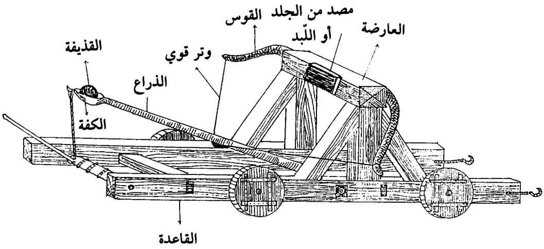
المنجنيق
