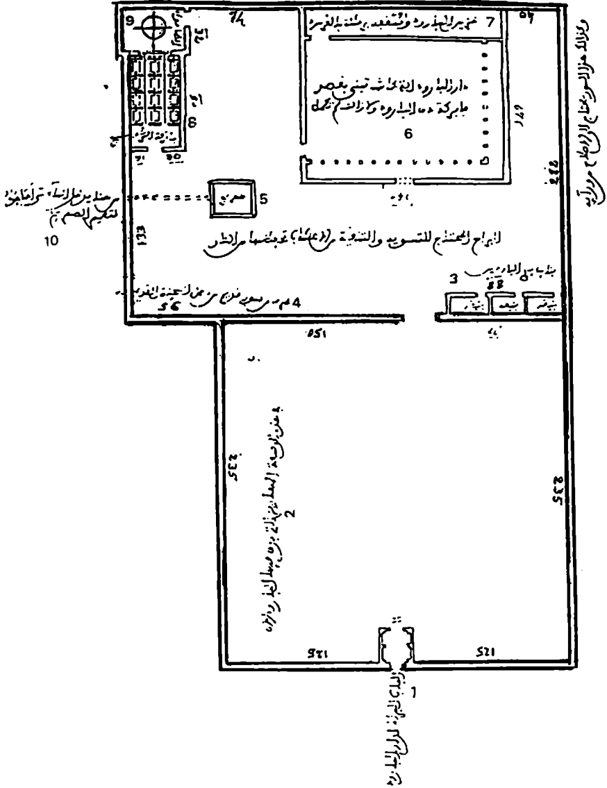
تصميم لمصنع البارود بمراكش (1)
