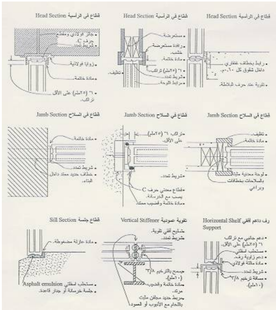
شكل رقم (٥٥) قطاعات تفصيلية لتركيبة الطوب الزجاجي بالحوائط
