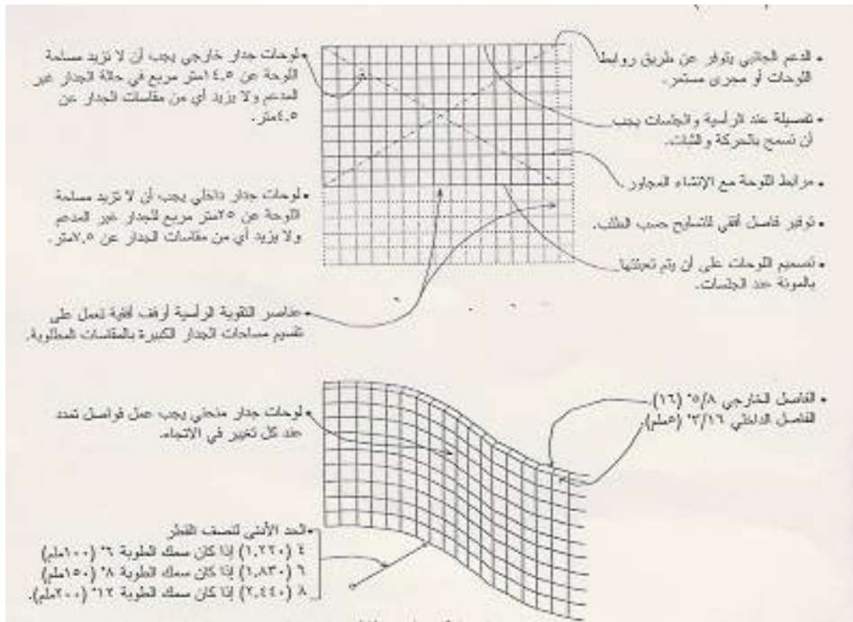
شكل رقم (٥٤) تفاصيل الشبكة التي تستخدم لتركيبة الطوب الزجاجي
