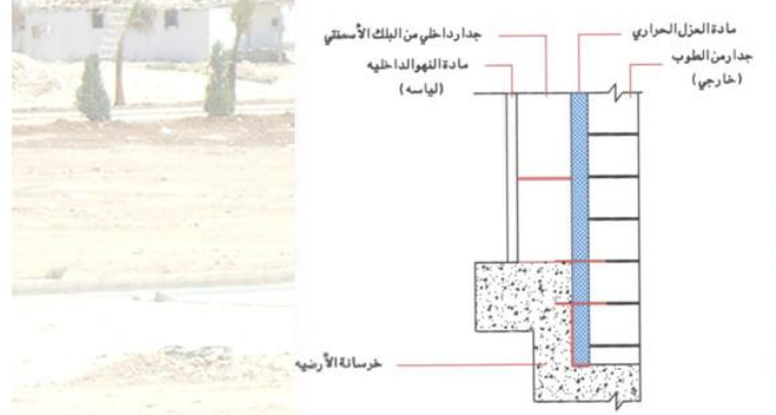
عزل حراري بين جدارين داخلي وخارجي
