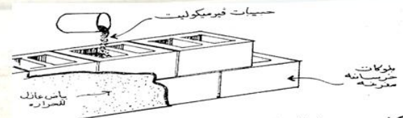
② طريقة العزل الحراري باستعمال الحبيبات السائبة
