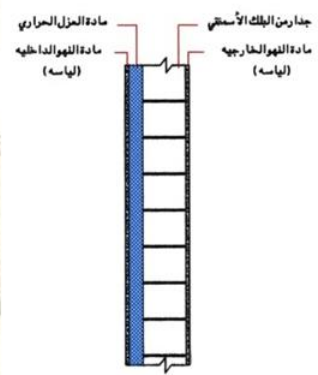
جدار معزول من الداخل
