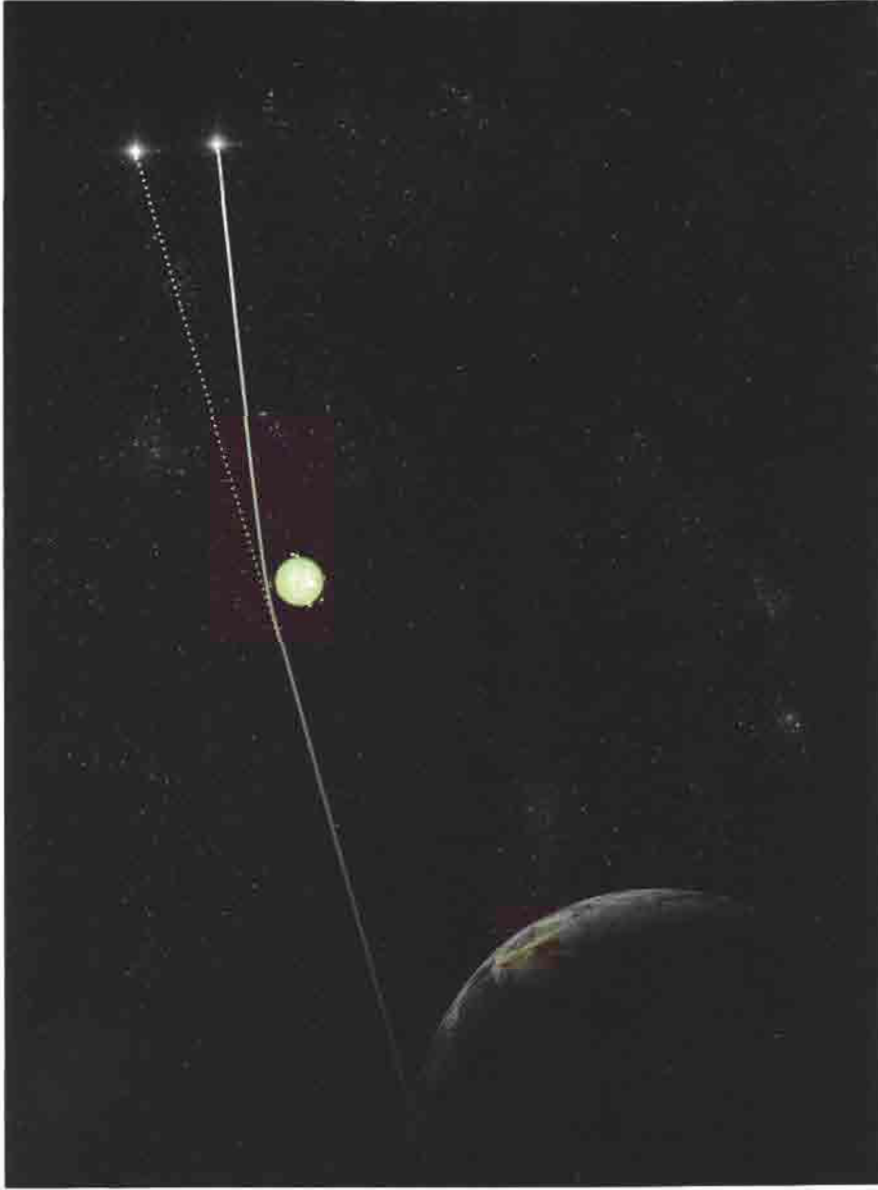
الحذاء الضوء بالقرب من الشمس عندما تقع الشمس مباشرة بين الأرض وأجرام بعيدة فإن مجال حاديتها يتسبب في انحاء الضوء فيؤدي إلى تحريف موقعه الظاهري
