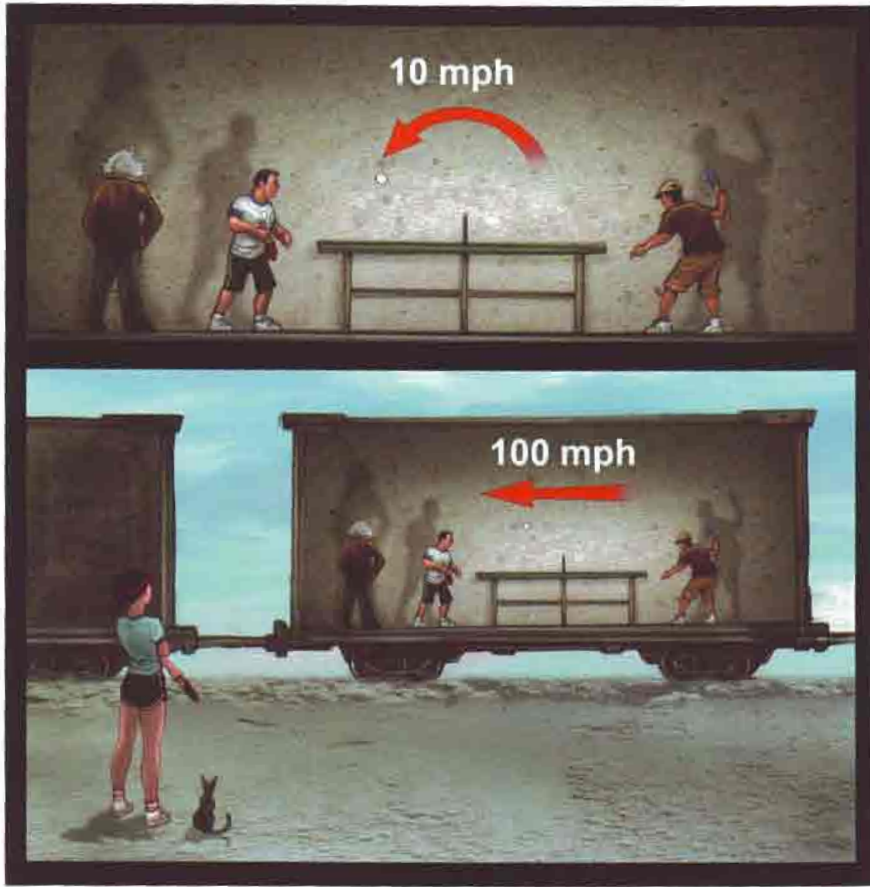
السرعات المختلفة لكرات نيس الضاؤنة وفقاً للنظرية النسبية فإن قياسات كل من مشاهد - على الرغم من اختلافها - صحيحة بالدرجة نفسها
