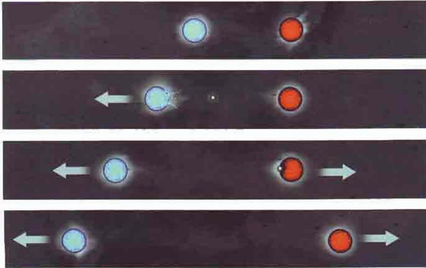
تبادل الجسيمات
