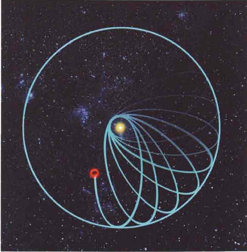
مسارات مدار عطارد
