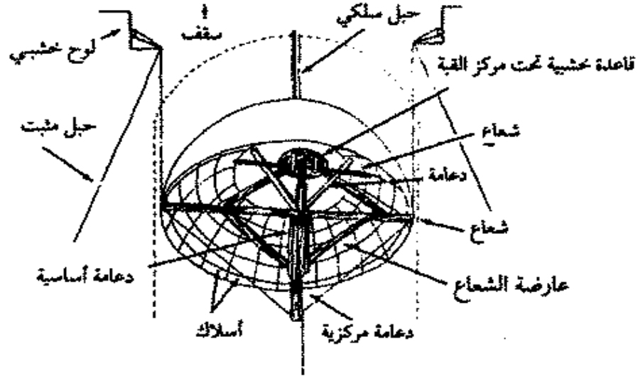
المبكل الخشبي ونظام البكرات الذي استخدم لانزال اللوحة - القبة في كنيسة ناكسوس
