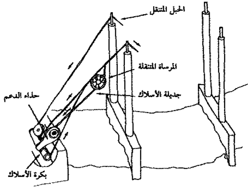
تعليق الكابلات الموازية فوق الجسر المعلق
