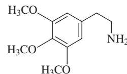
Mescaline
