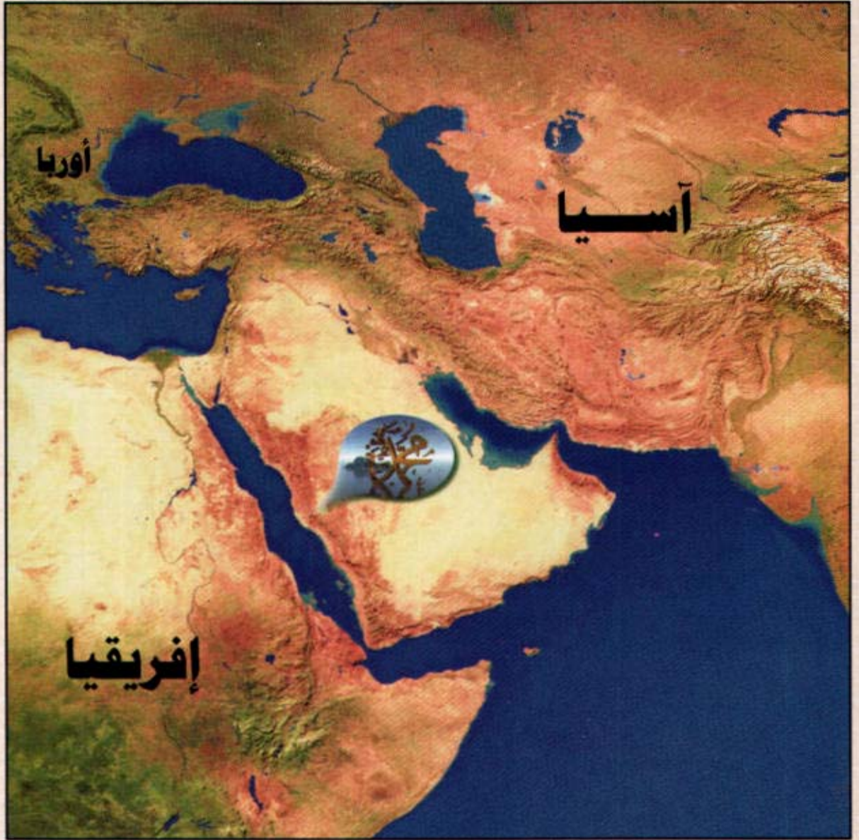
الخريطة الطبيعية لغرب قارة آسيا وشرق إفريقيا
