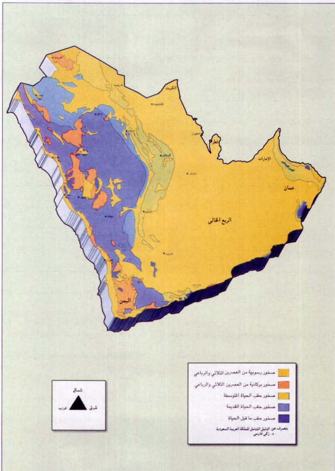
الهيكل الجيولوجي لشبه الجزيرة العربية
