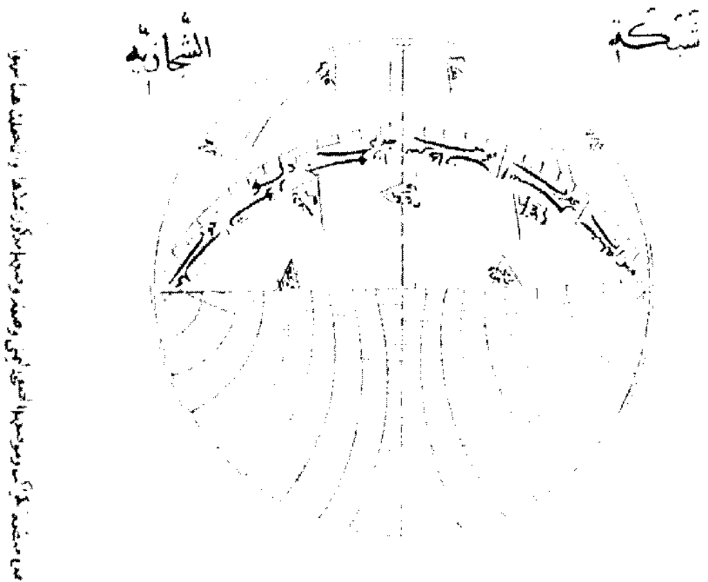
الشكل (٩:٨): يوضح شبكة أسطرلاب آفاقي وردت في رسالة ابن السراج عن الآلات الفلكية (مخطوطة مكتبة شيلستر بيتي بدبلن، رقم ١٠٢)
