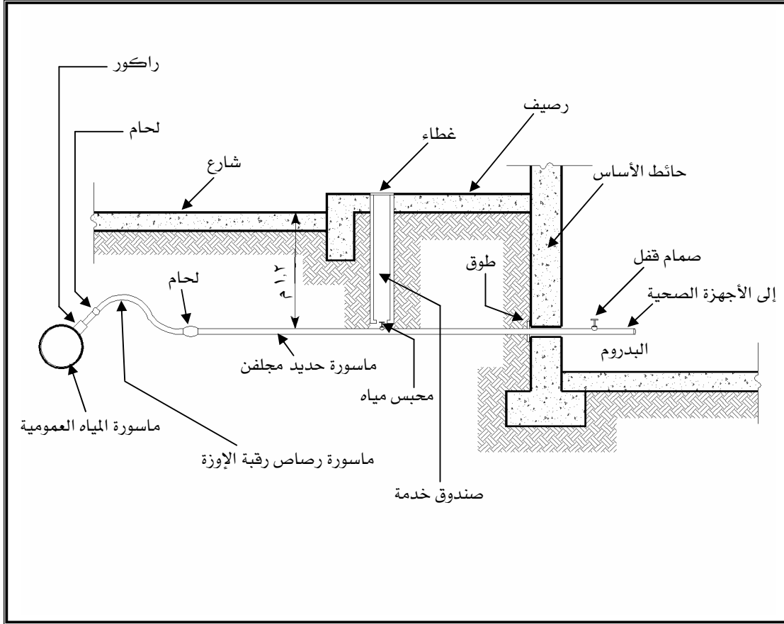
شكل (١- ٢٢) : توصيل المياه للمبنى في حالة أن ماسورة التغذية من الحديد المجلفن
