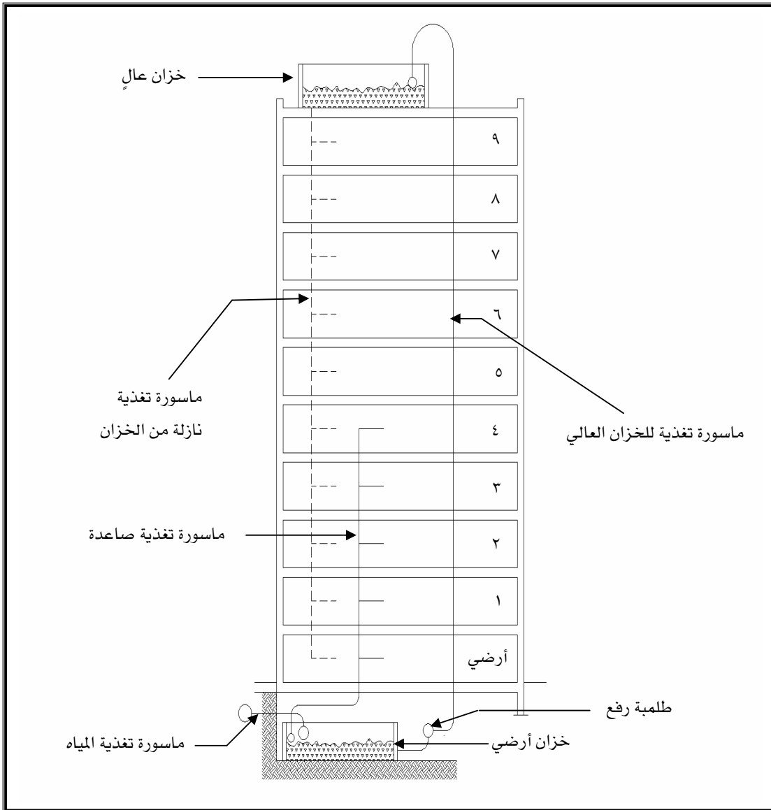
شكل (١ - ٣٠) : التغذية بتجميع ضغط الشبكة و ضغط الخزان و الرفع بطلمبات للخزان العالي من خزان أرضي و تغذية الأدوار المنخفضة بضغط الشبكة
