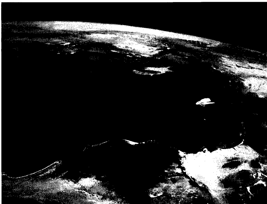
صورة من أحد الأقمار الصناعية لدلتا النيل على البحر الأبيض المتوسط
