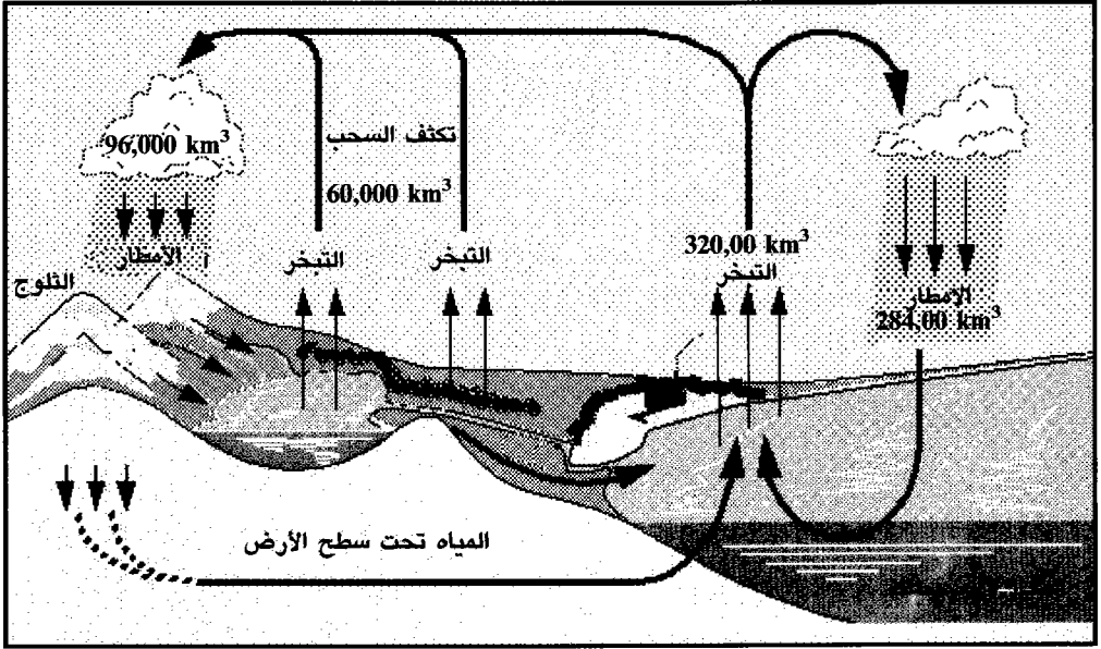
رسم تخطيطي لدورة الماء حول الأرض
