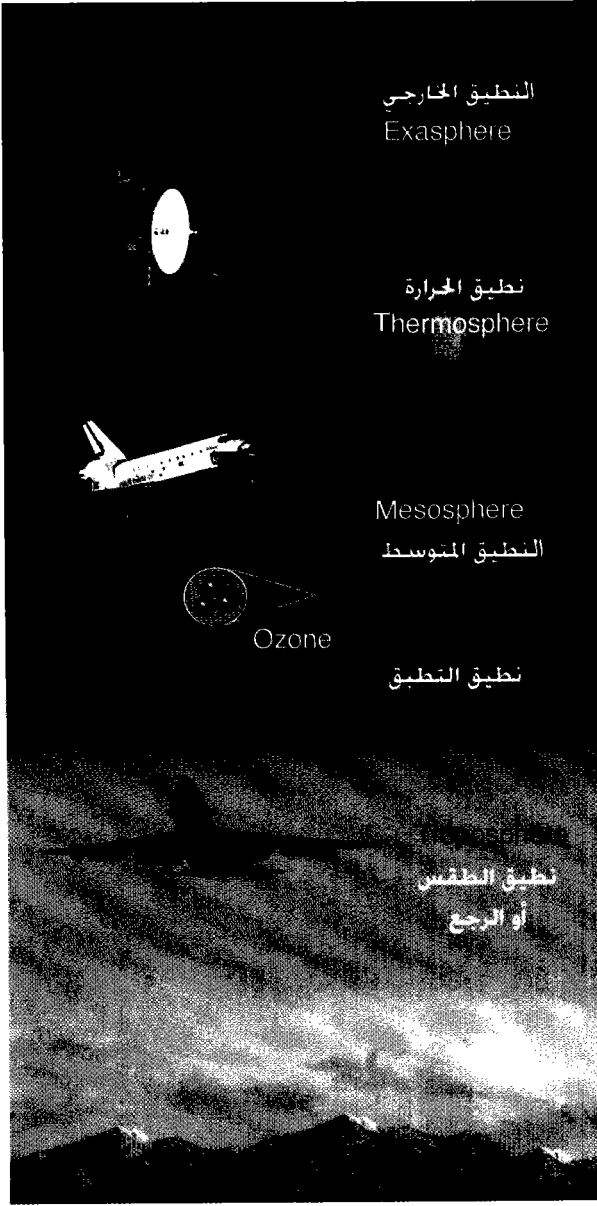
رسم تخطيطي لتكوين الغلاف الغازي للأرض
