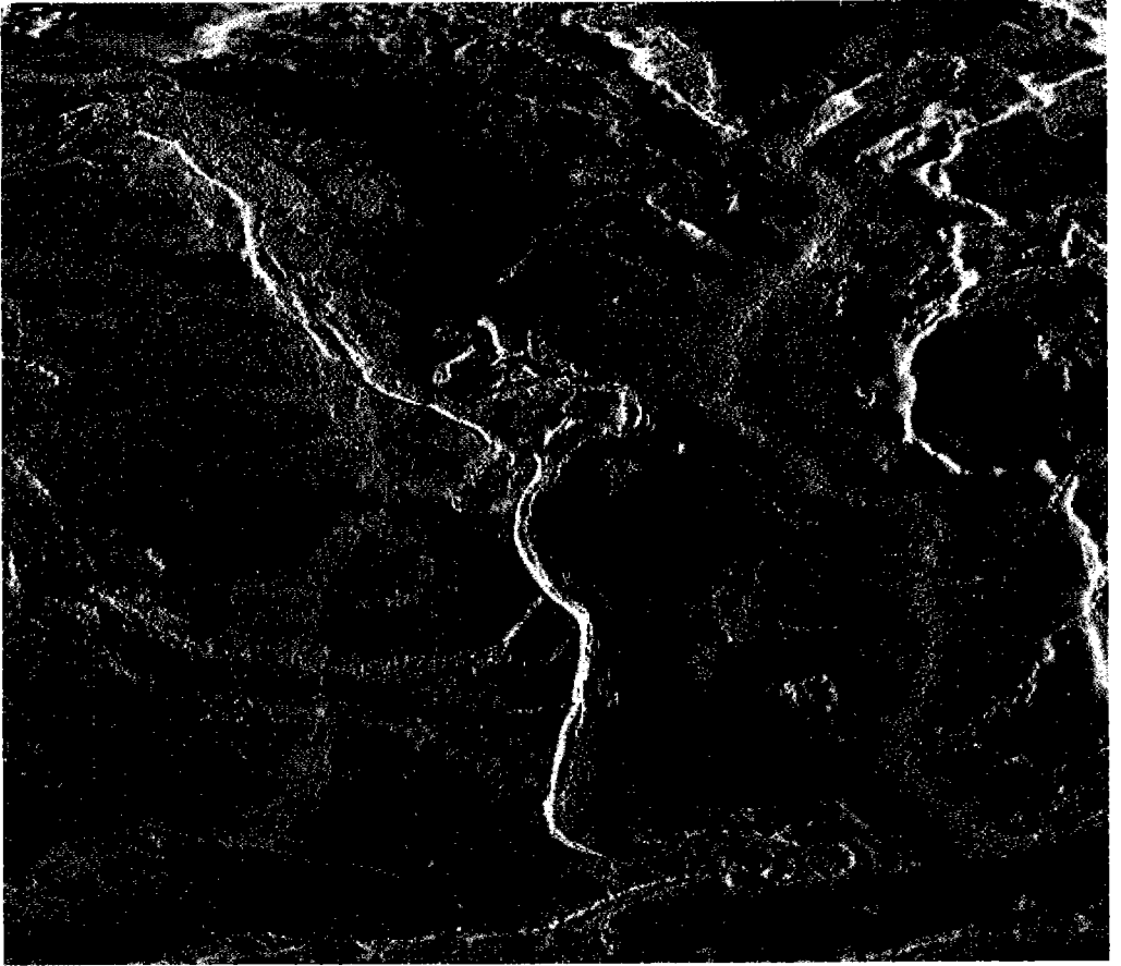
رسم يوضح تصدع قيعان المحيطات بشبكة متصلة من الصدوع وتكوّن سلاسل جبال أواسط تلك المحيطات (حيود أواسط المحيطات)
