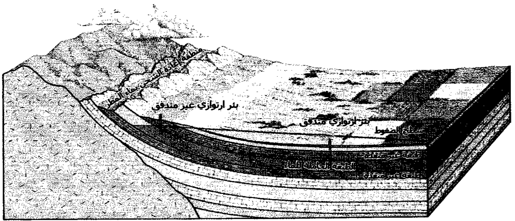
رسم لحركة الماء وخزونه داخل قشرة الأرض
