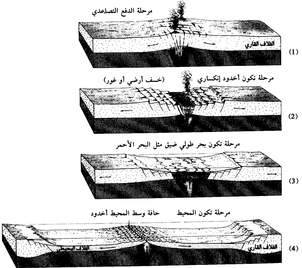
شكل يوضح مراحل تكون المحيطات عن طريق تكون الخسوف الأرضية
