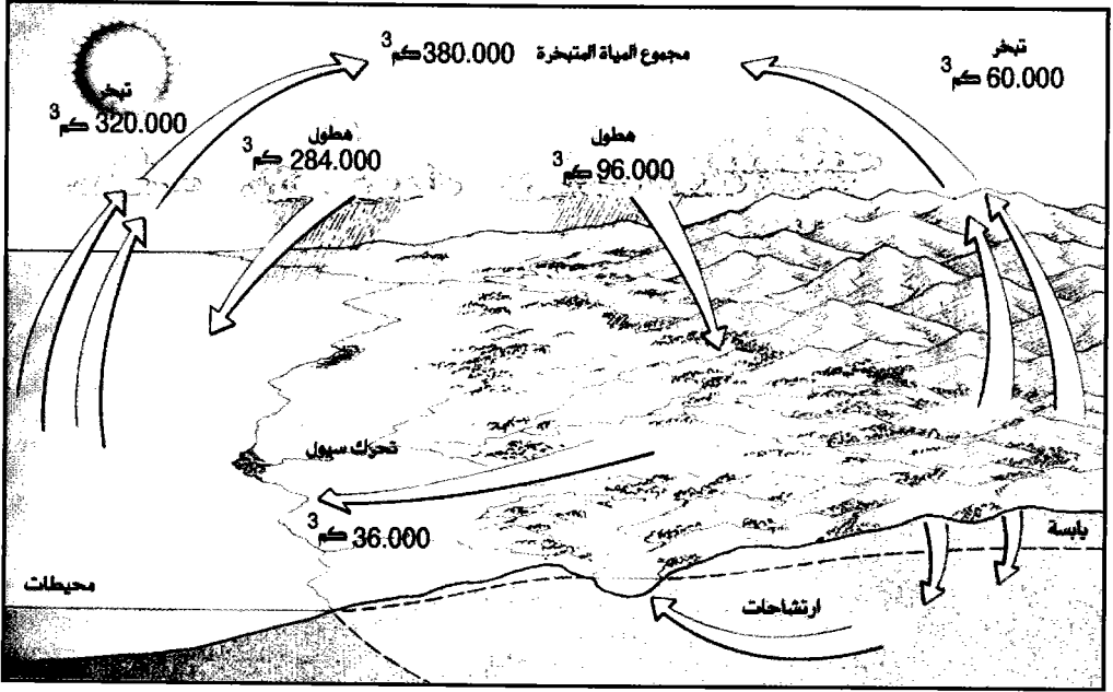
رسم تخطيطي يوضع دورة الماء حول الأرض
