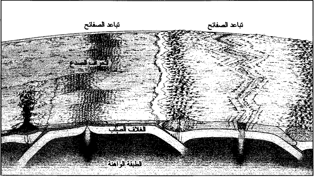
صورة لتحرك ألواح الغلاف الصخري للأرض
