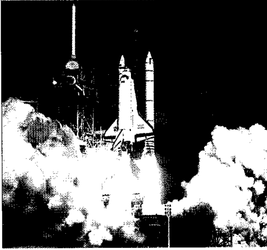
صورة للمركبة الفضائية «ديسكفري» لحظة انطلاقها
