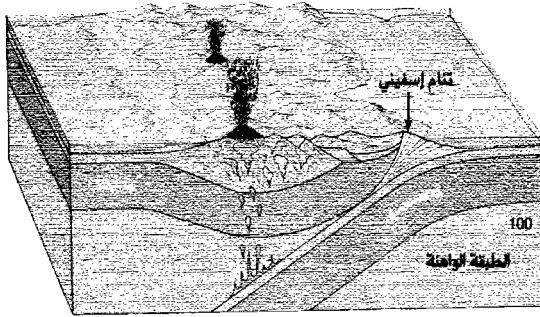
قوس جزري مكتمل
