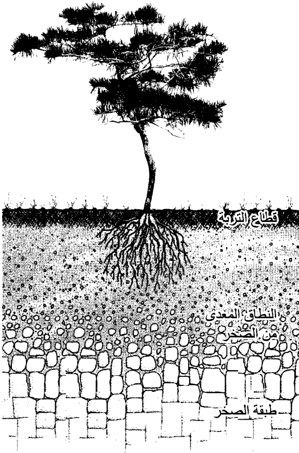
رسم تخطيطي لقطاع التربة يوضح نطاقها الأربعة
