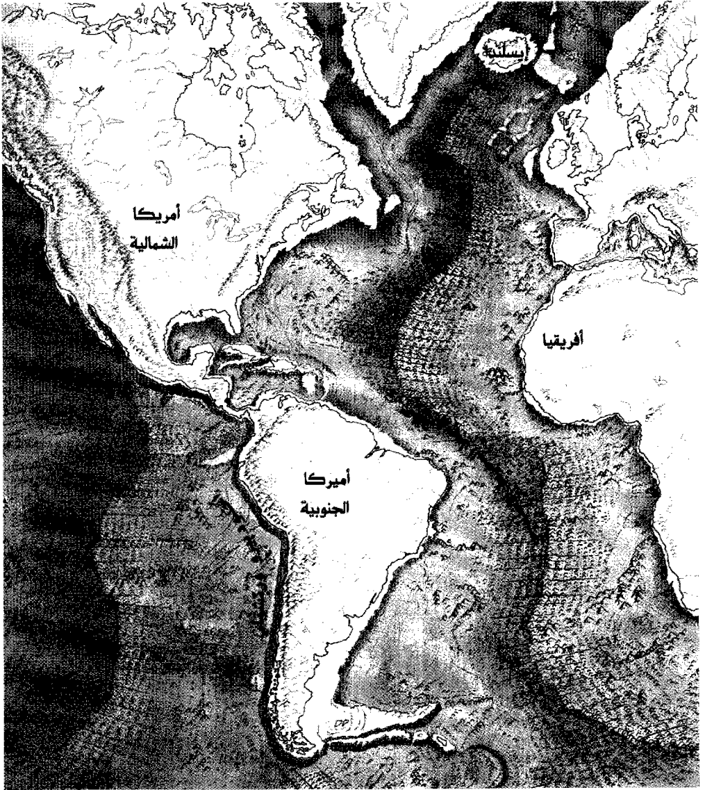
خارطة توضح حواف أواسط المحيطات والأخاديد الناتجة عن نزول قيعان المحيطات تحت القارات
