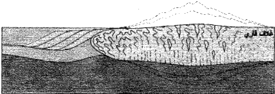
رسم يوضح حركة بروز الجذور كلما برت عوامل التعرية قمم الجبال
