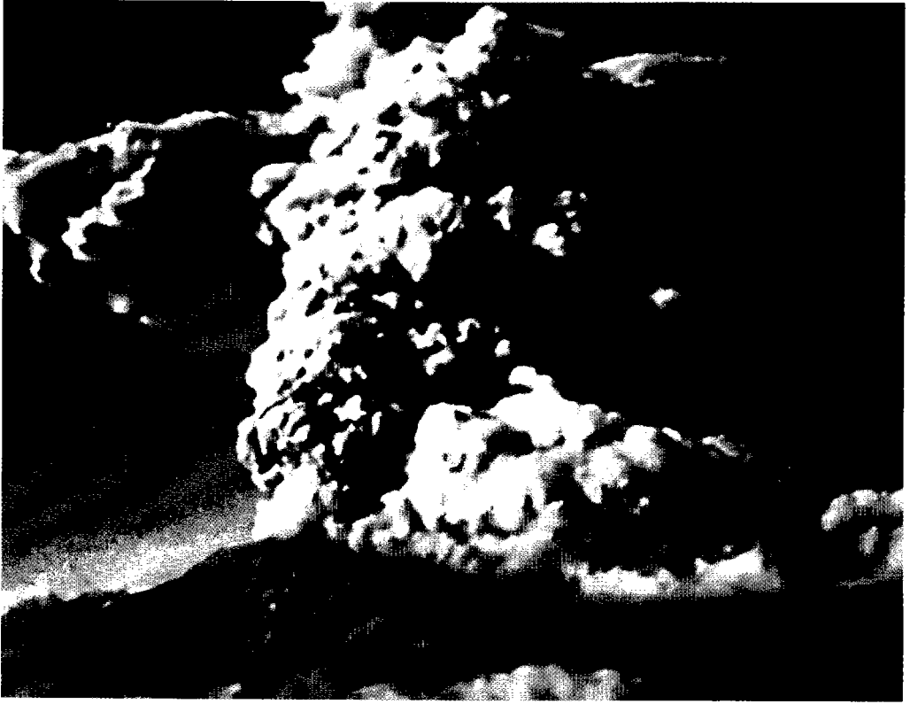
سحب بركانية ضخمة تتصاعد من بركان سانت هيلين بولاية واشنطن سياتل
