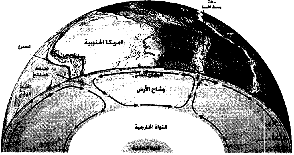
رسم قطعي للكرة الأرضية يظهر نطق الأرض الداخلية وحركاتها، وتأثيرها على السطح
