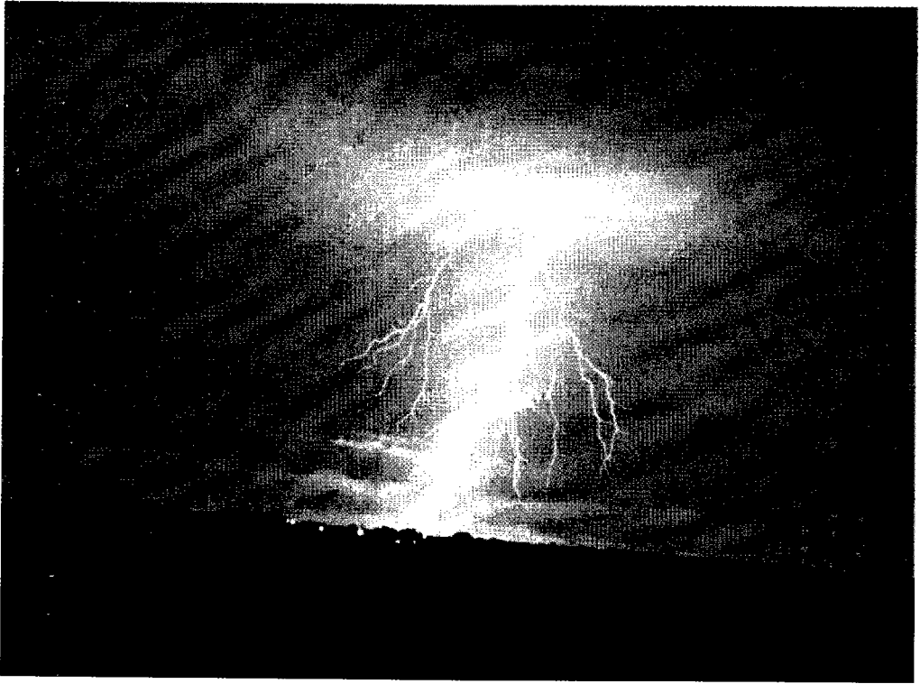
صورة للبرق الذي يحدث في نطاق المناخ (بين السماء والأرض)
