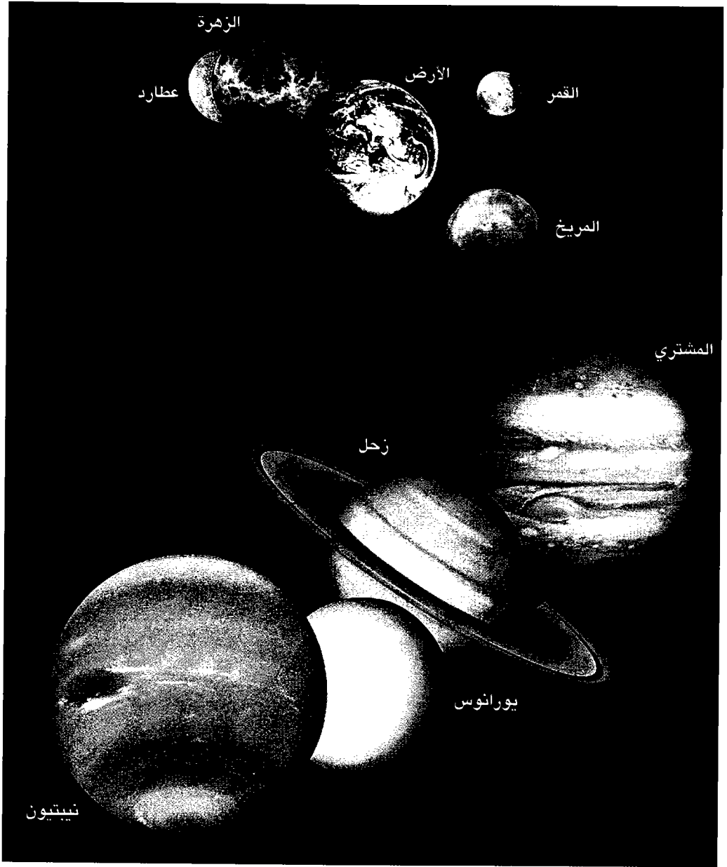
صورة حقيقية لكواكب المجموعة الشمسية التقطتها سفينة الفضاء «فويديجر - 1» من خلف مدار كوكب نبتون (Voyager-1 Photograph for the Planets of our Solar System)
