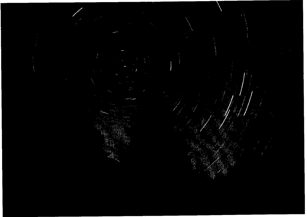
صورة في المنطقة الشمالية القطبية تبين ثبات النجم القطبي (تصوير بطيء)
