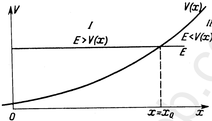
الشكل ١ - ٥ . توضيح حل المعادلة الموجية بطريقة W.K.B.
