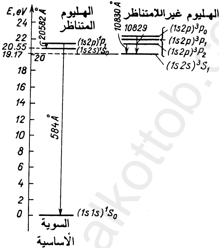
الشكل ٢٤ - ٢. مخطط سويات الطاقة في ذرة الهليوم . الانشطار للسويات - ^3P معطى بمقياس الرسم ، طول الموجة مقدر بالانجستروم ( \text{Å} ) ، حيث 1 \text{ Å} = 10^{-8} \text{ cm} .
