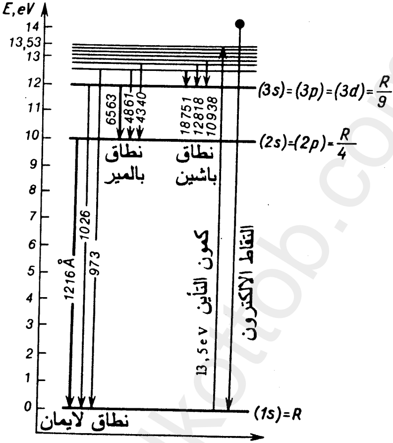
الشكل ١٢ - ٣. النطاقات ( السلاسل ) الطيفية لذرة الهيدروجين ، أطوال الموجات المقابلة للانتقالات المبينة مقدره بالـ \text{\AA} .
