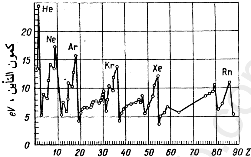
الشكل ٢٧ - ١ . تابعة طاقة التأين للرقم الذري من أجل ذرة معتتلة .
