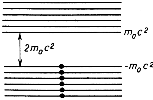
الشكل ٢٢ - ٢. مخطط طاقة الصفر لفرغ الكترون - بوزيترون .
