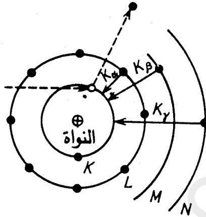
الشكل ٢٥ . مخطط ظهور الطيف المميز ( طبقا لكوسيل ) ، . الكترونات ، أما الخط المتقطع فيبين عملية ترك الالكترون للغمامة - K .
