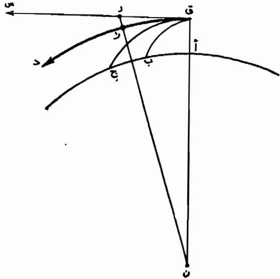
الشكل ١٤ - المقطوع لذي تسقطه في ثانية قذيفة مندفة بسرعة كافية لأن لا تهبط في ب ارج بل لأن تدور حول الارض وفقاً لدائرة شعاعها ن ق .
