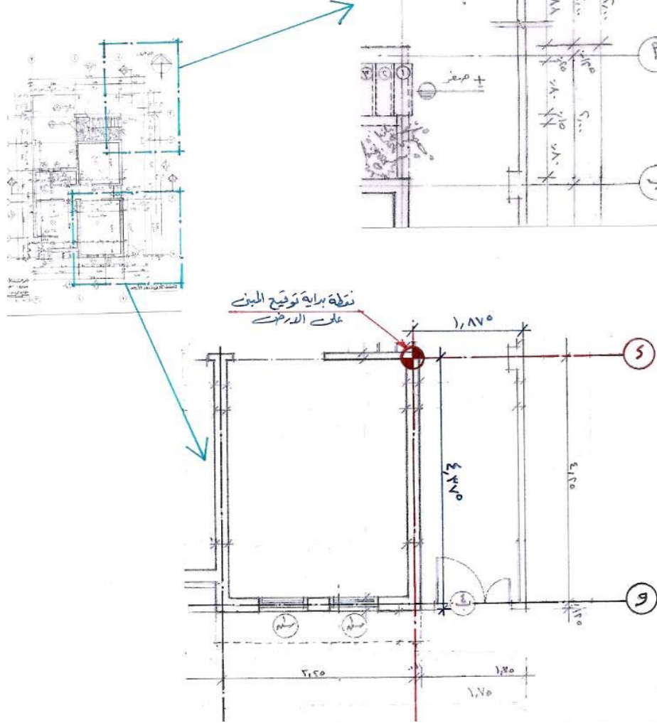
شكل رقم " ١١ " المعلومات الأساسية بلوحة المسقط الأفقي التنفيذي ( وضع المحاور، وتحديد نقطة بداية توقيع المبنى على الأرض )
