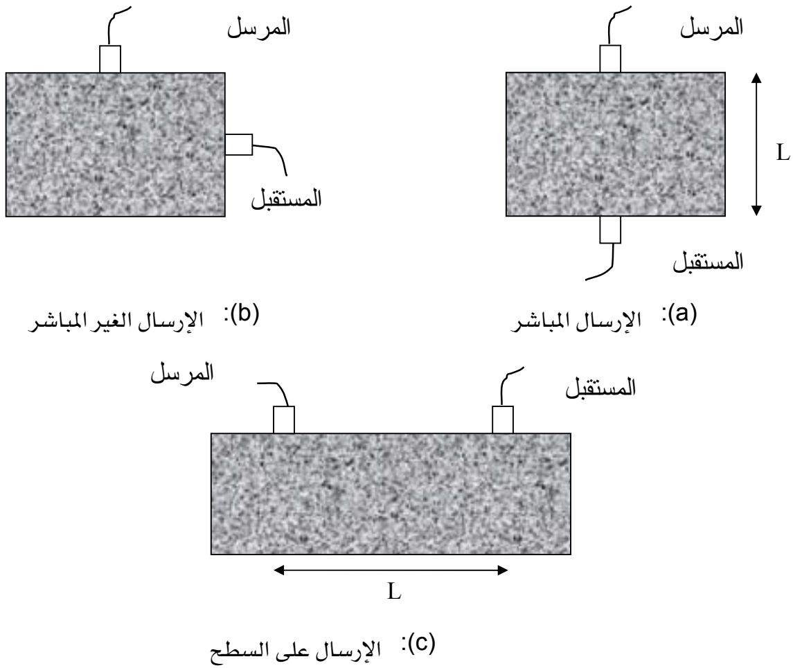
شكل رقم ١٤,٧ : طرق الإرسال و الاستقبال موجات فوق الصوتية.
