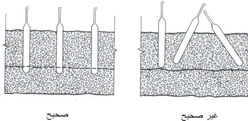
شكل رقم ١٤,١:الوضعية الصحيحة للهزاز الداخلي لتكثيف الخرسانة.
