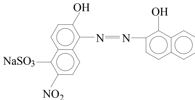
الشكل ٥: التركيب الكيميائي لدليل إريوكروم بلاكتي Eriochrome black T
