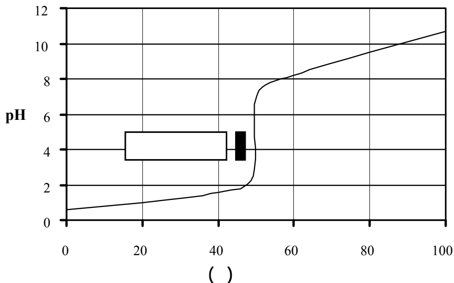
الشكل ٣: منحنى معايرة حمض قوي بقاعدة ضعيفة
