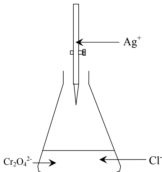
الشكل ١: طريقة موهر Mohr's method.
