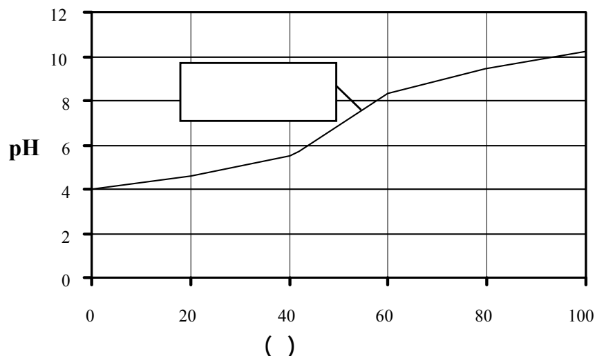
الشكل ٤: منحنى معايرة حمض ضعيف بقاعدة ضعيفة
