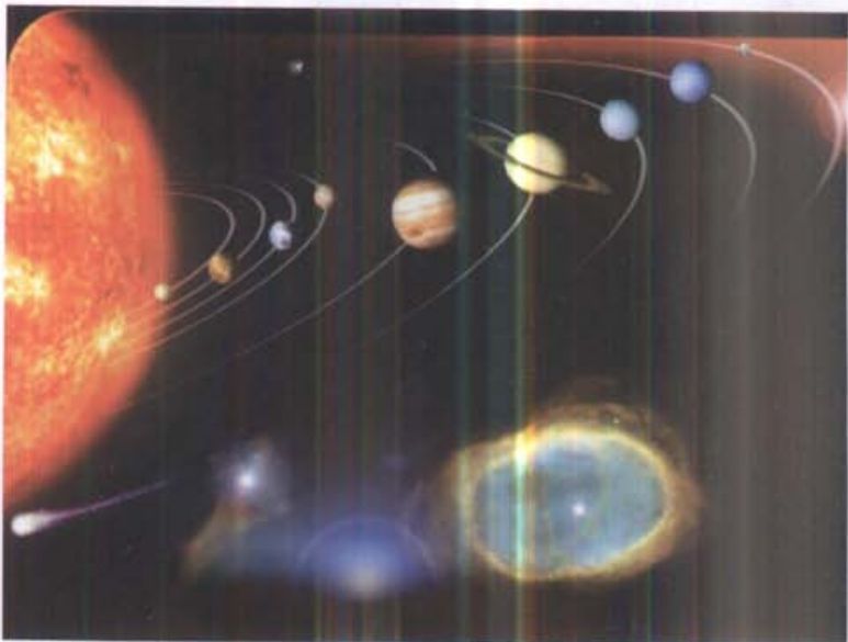
نظام شمسی
