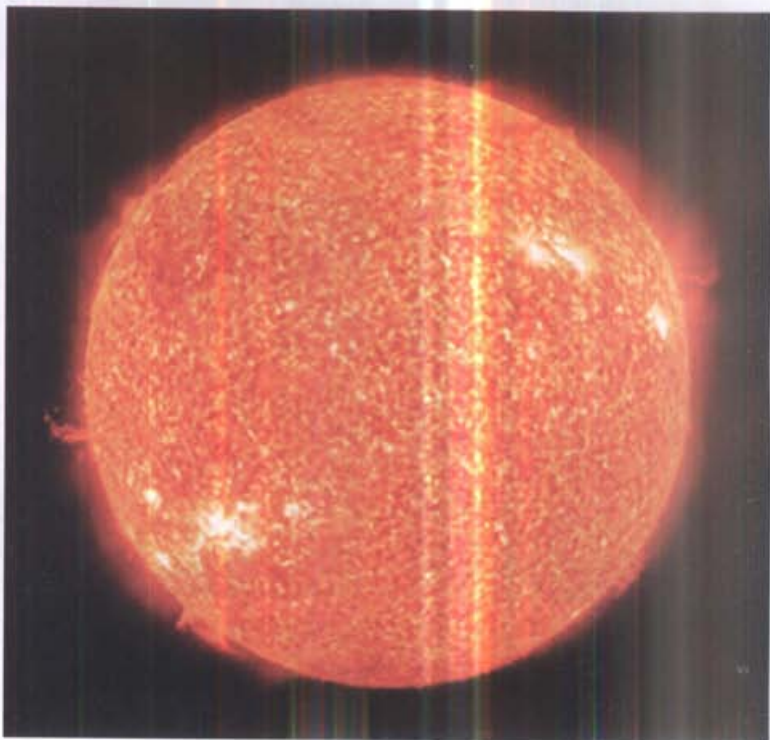
Sun
