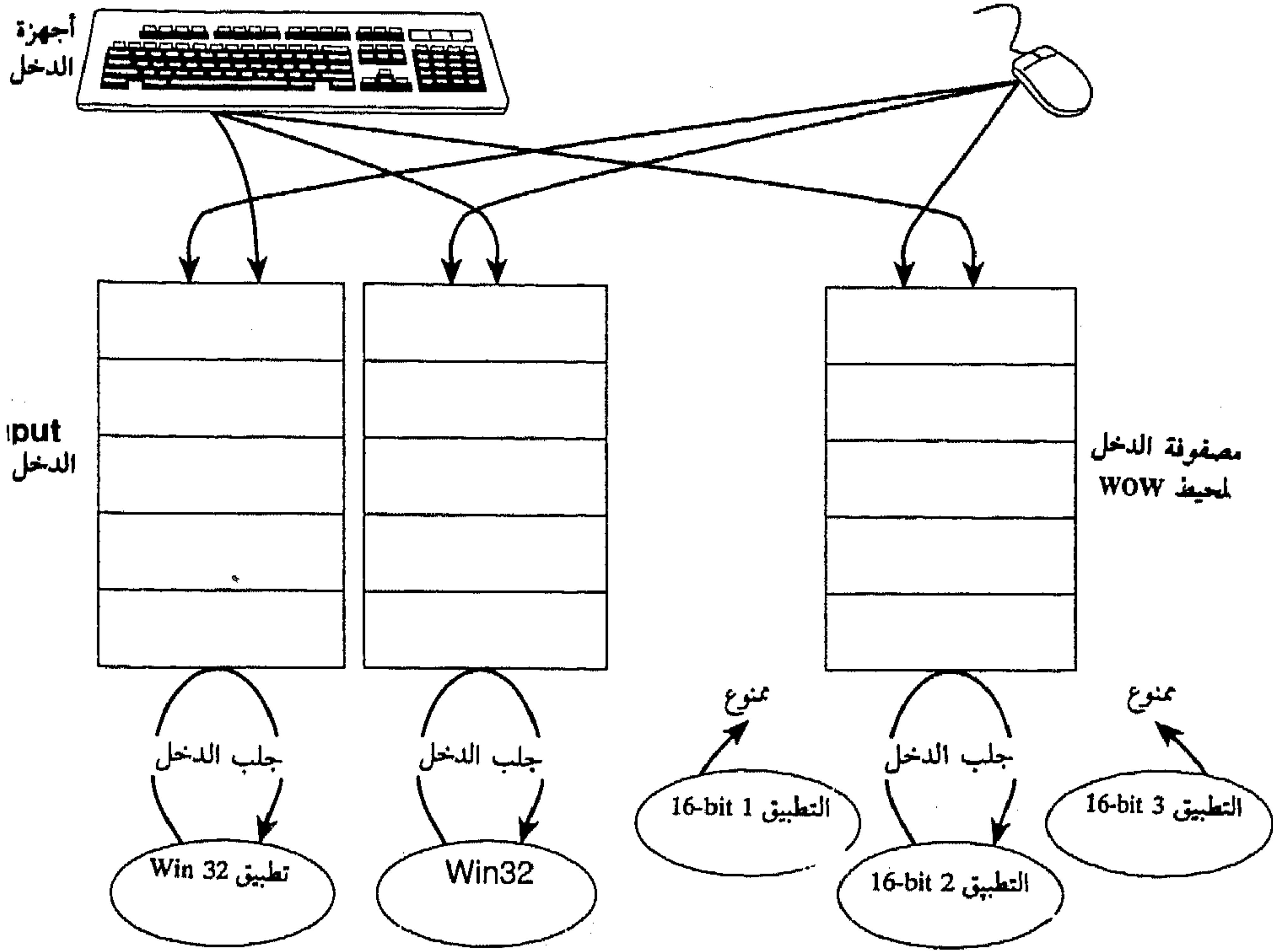
الشكل (18-5) نموذج الدخول لمحيط WOW
