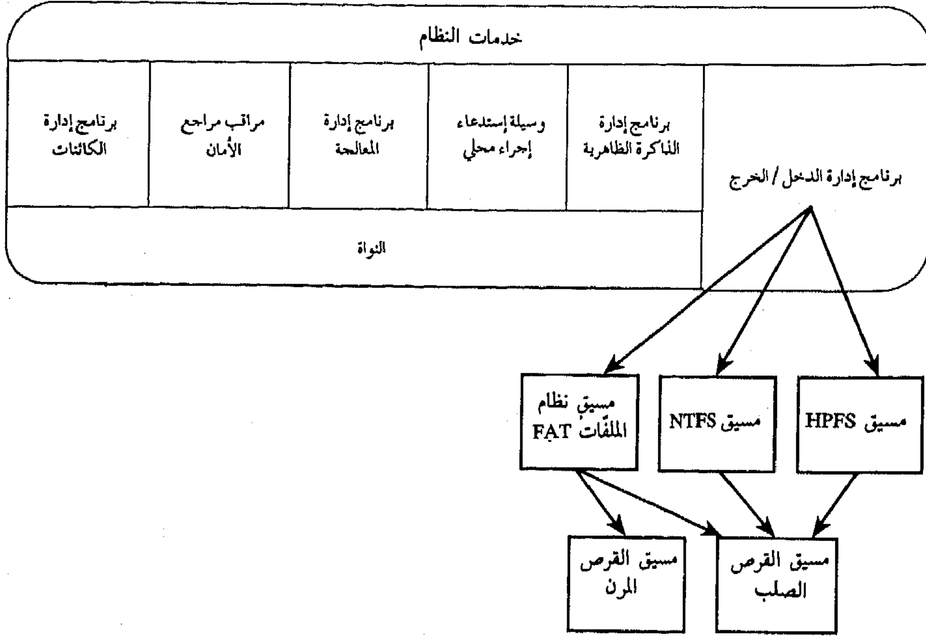
الشكل (14-2) المسقات المرتبة في طبقات
