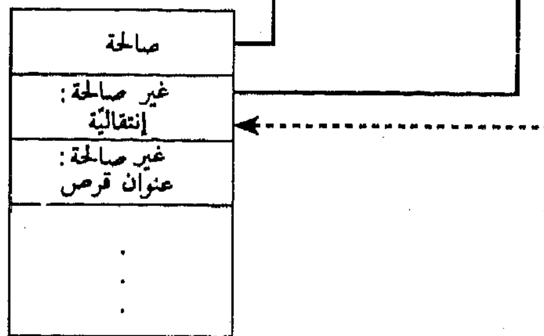
جدول صفحات المعالجة 3
