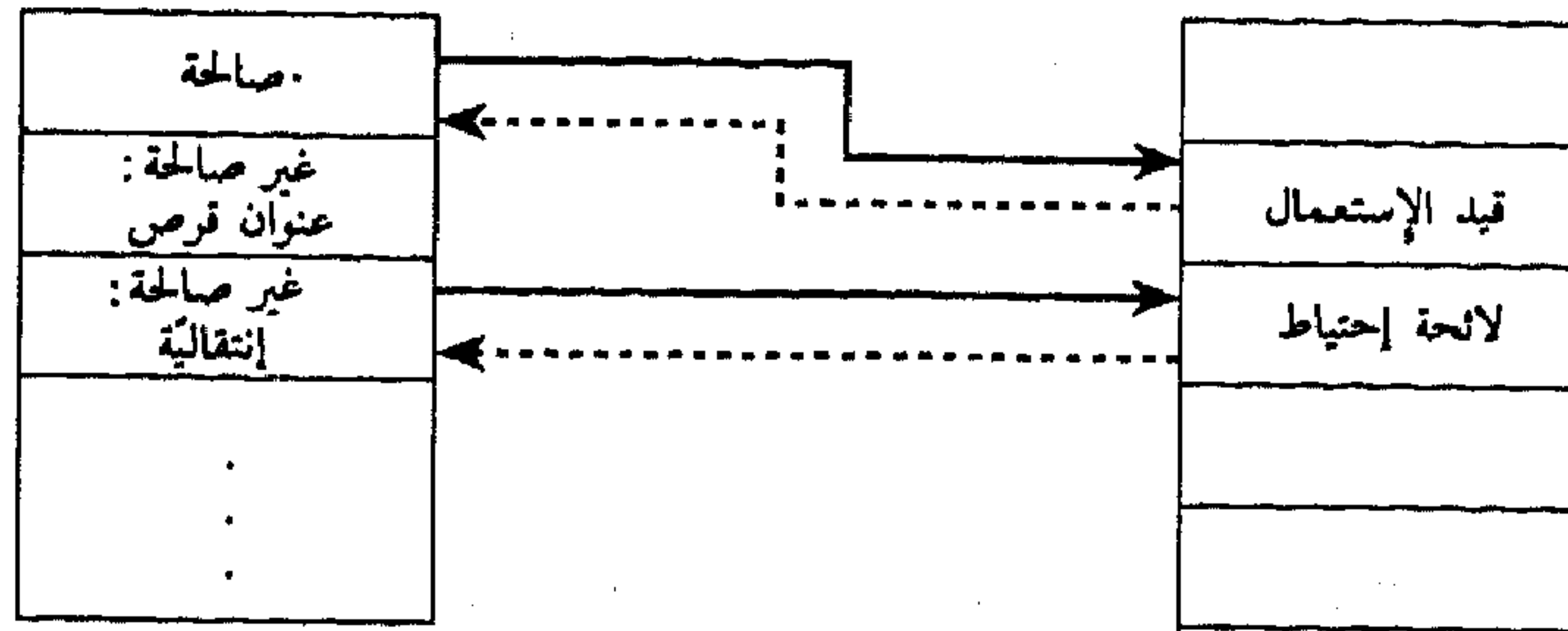
قاعدة بيانات إطار الصفحة
