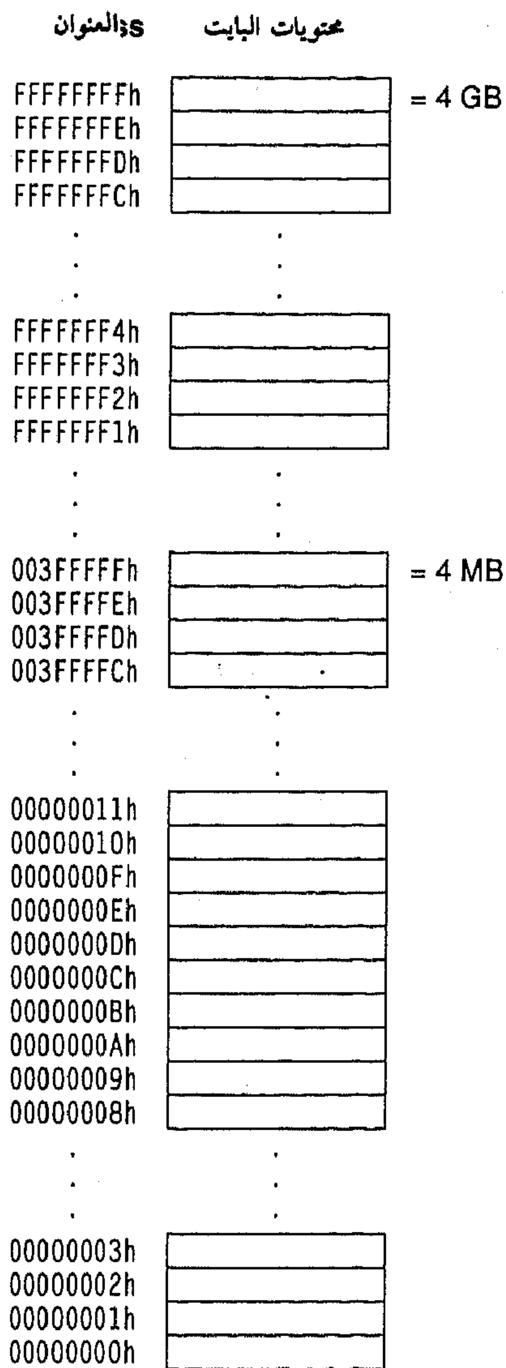
الشكل (2-6) فسحة العنوان الظاهري الخطي
