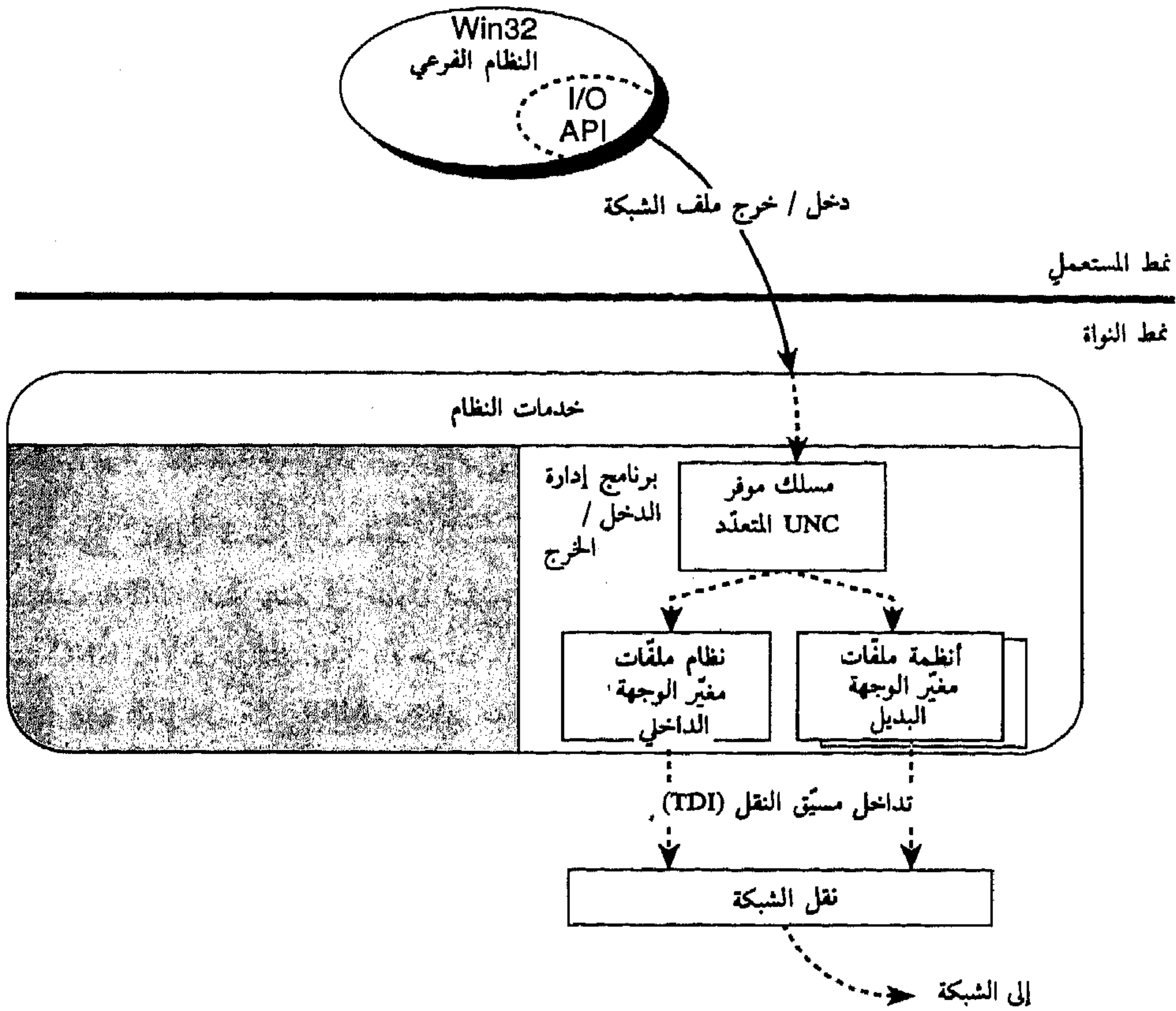
الشكل (11-9) موقر UNC المتعمد (MUP)
