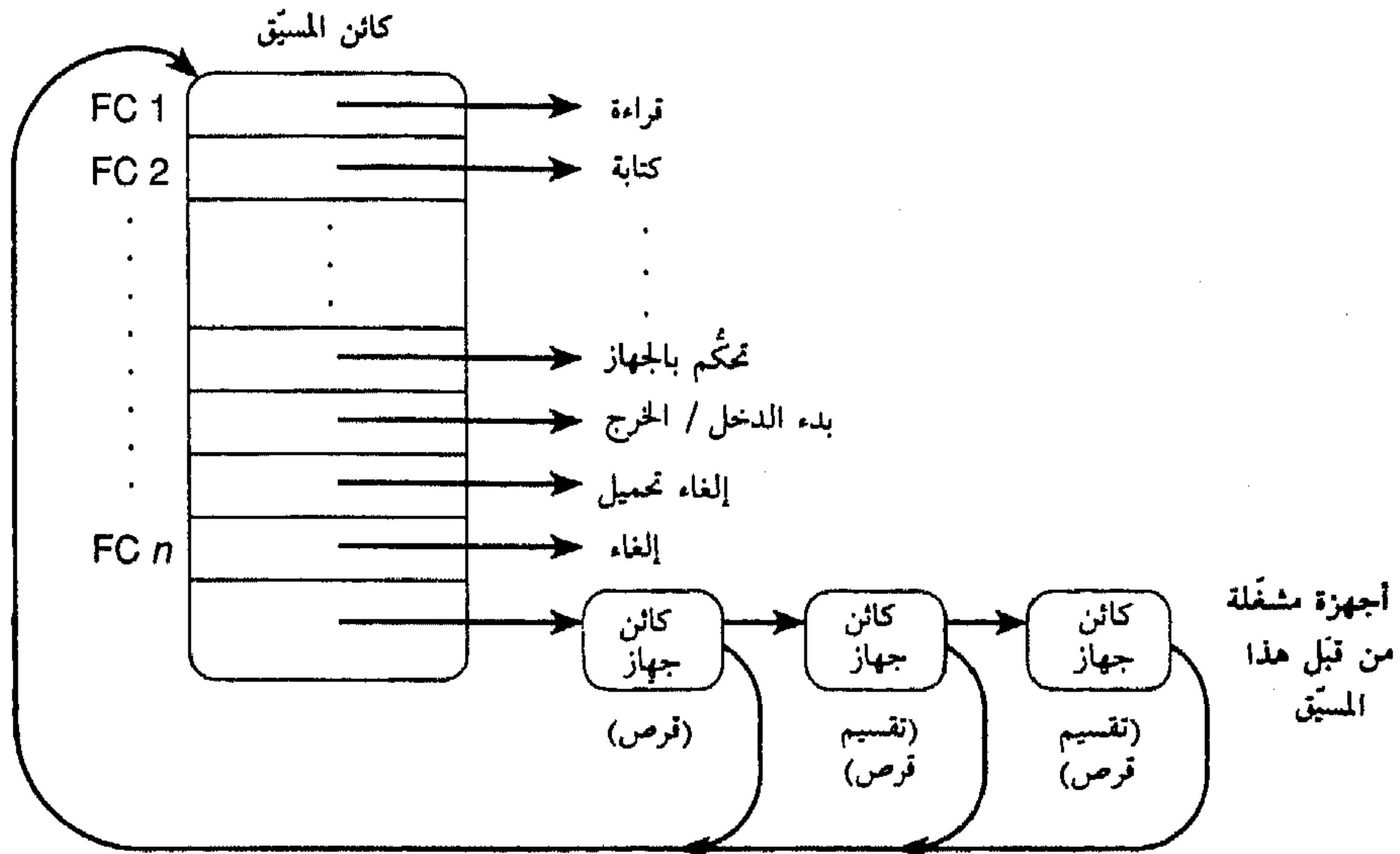
الشكل (8-20) كائن المسيق
