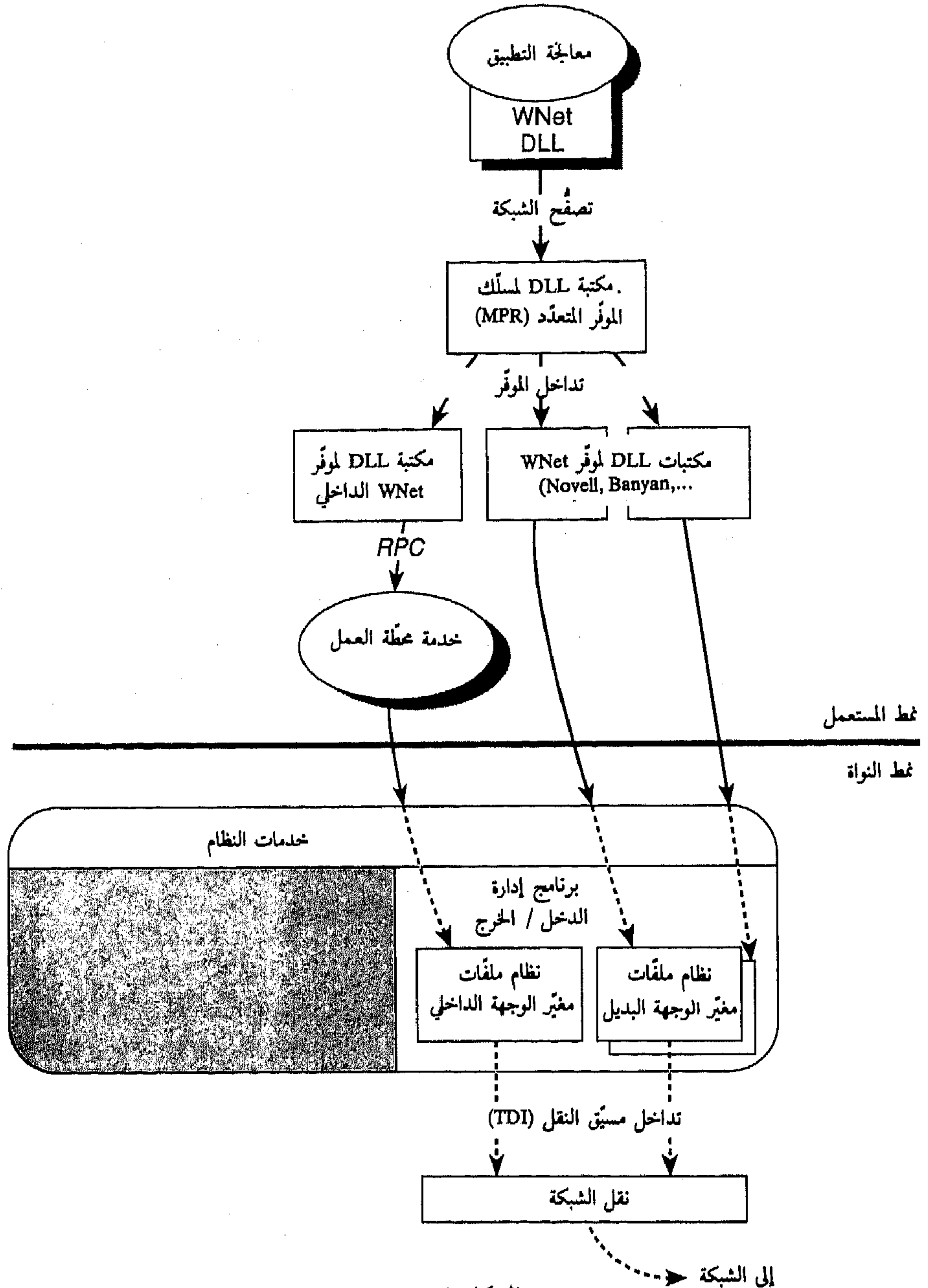
الشكل (9-9) برامجيات الموفر المتعدد
