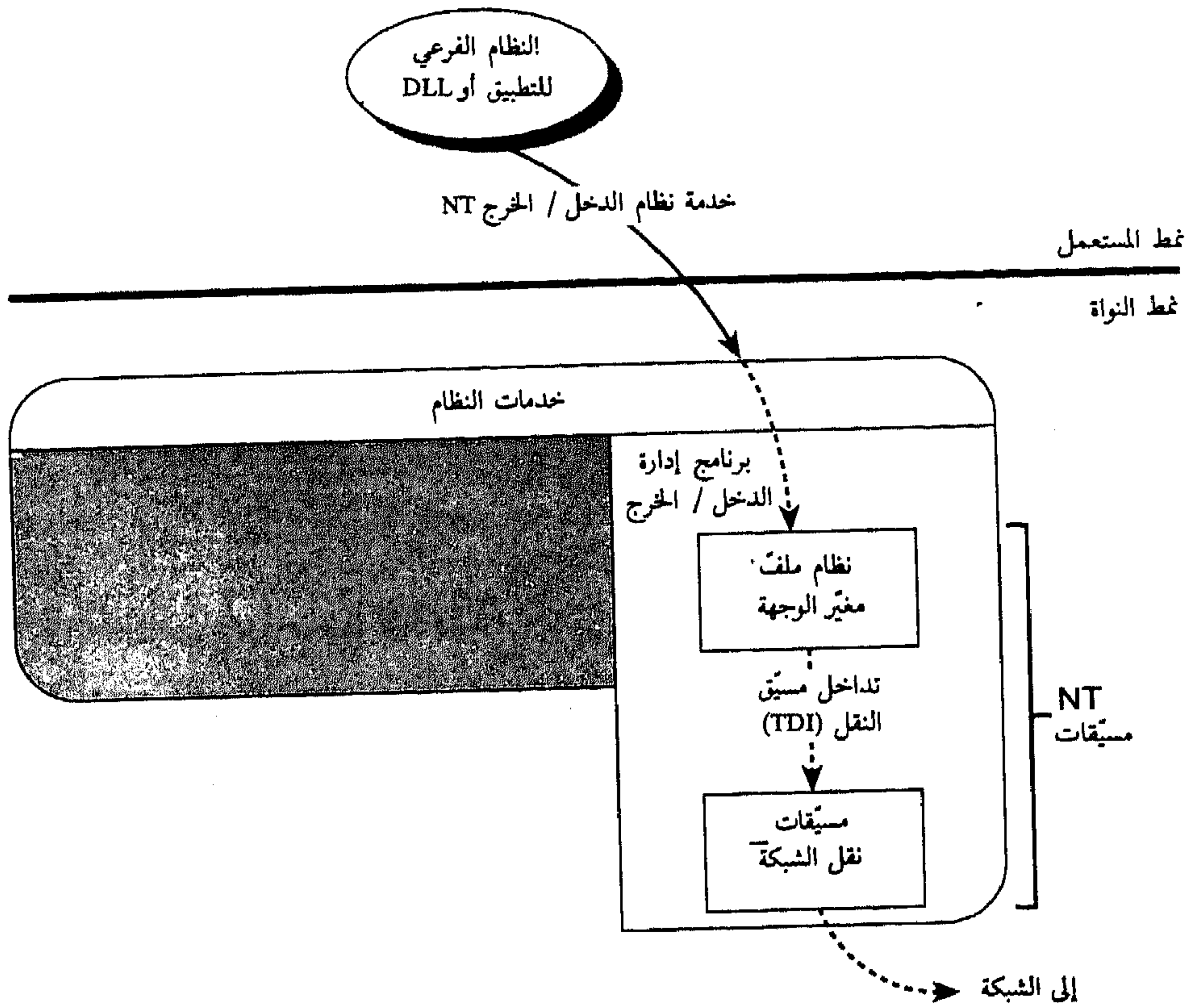
الشكل (3-9) معاينة شبكة الدخول / الخرج المبسطة من جهة المستضاف
