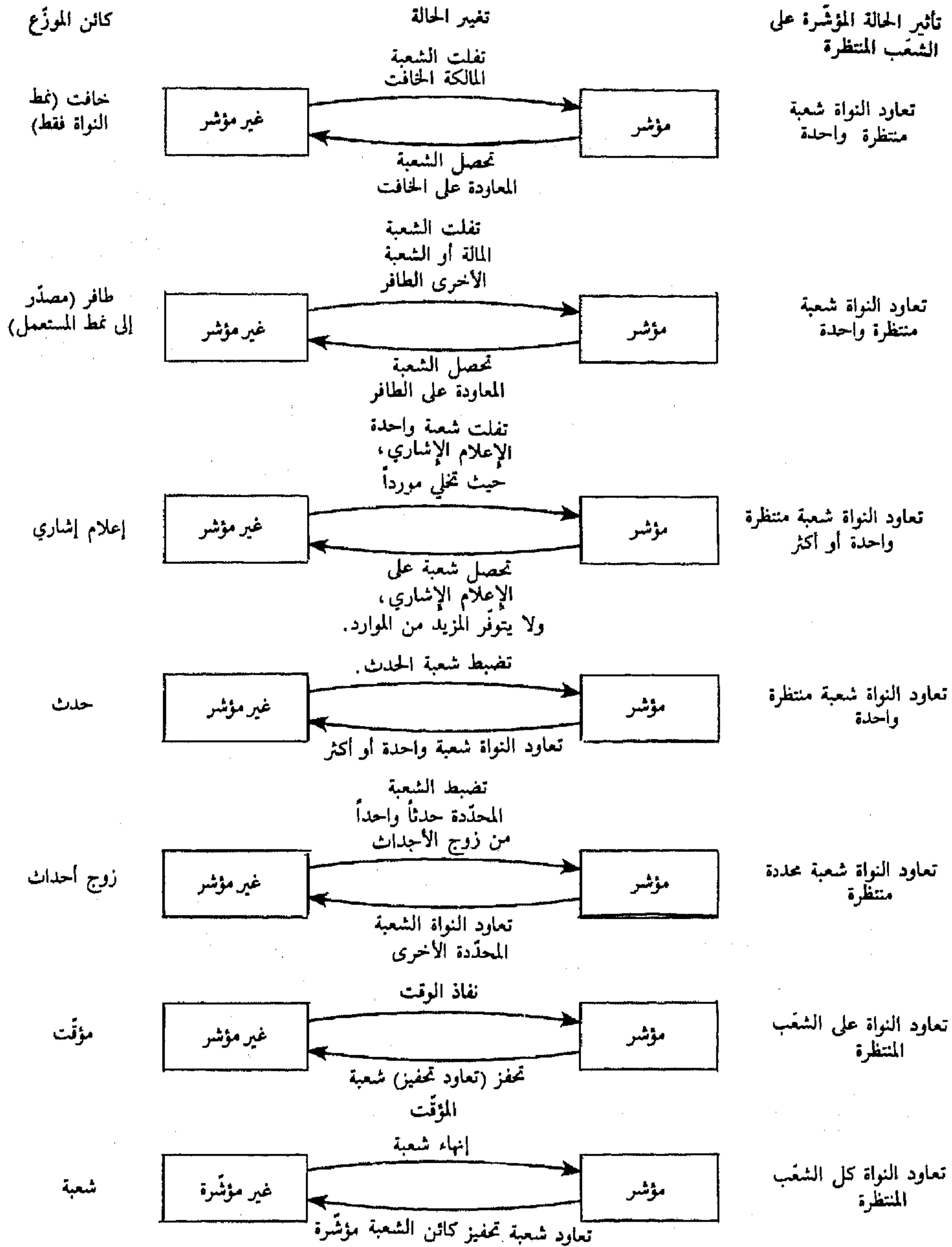
الشكل (15-7) كائنات موزع النواة المنتقاة
