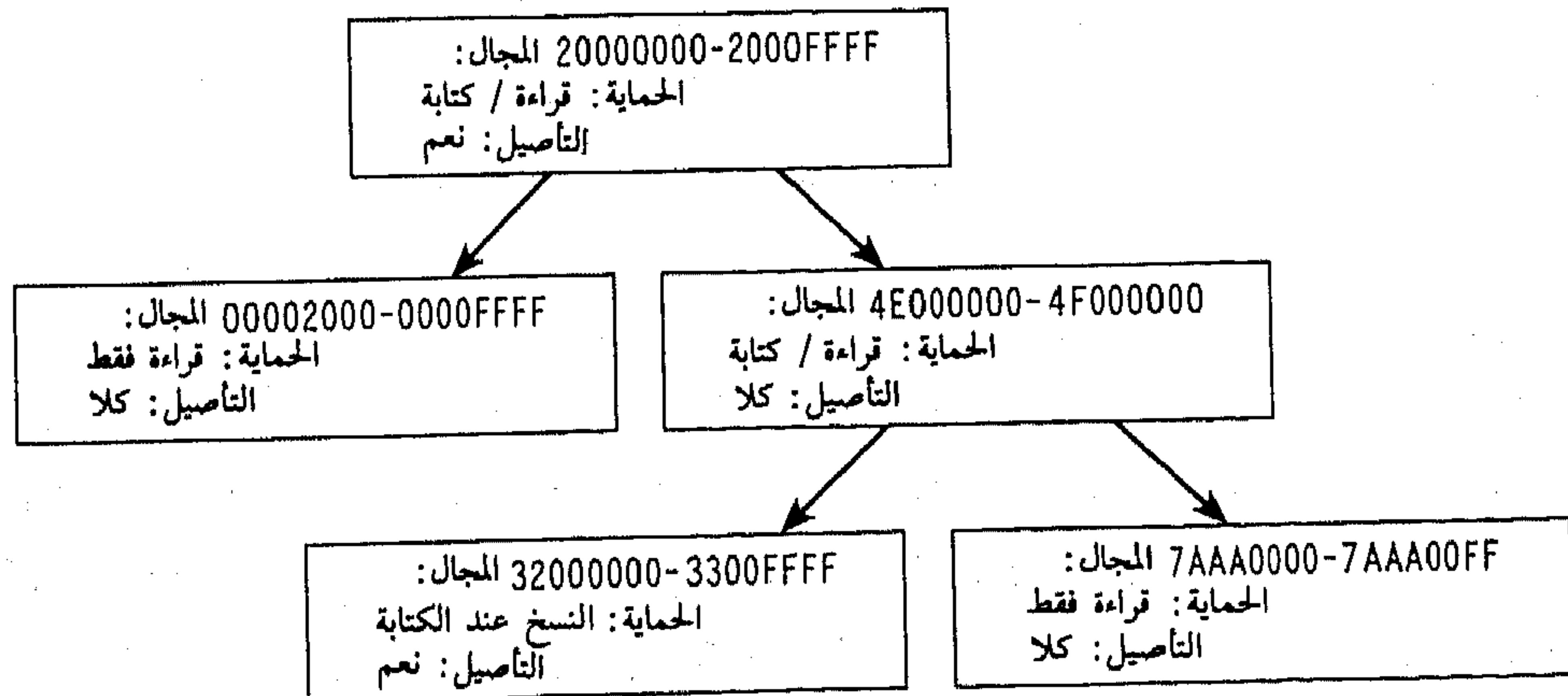
الشكل (6-16) واصفات العنوان الظاهري
