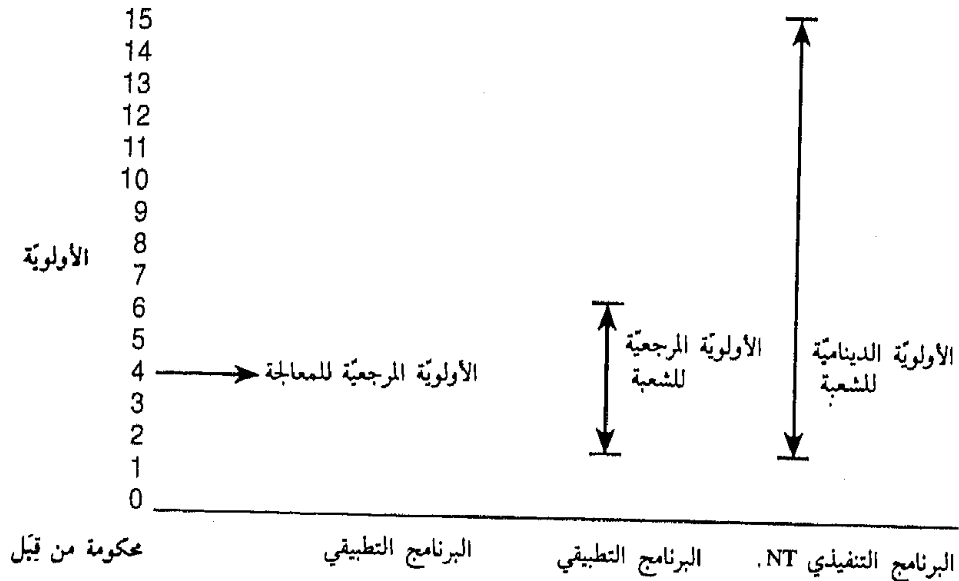
الشكل (10-4) علاقات الأولوية
