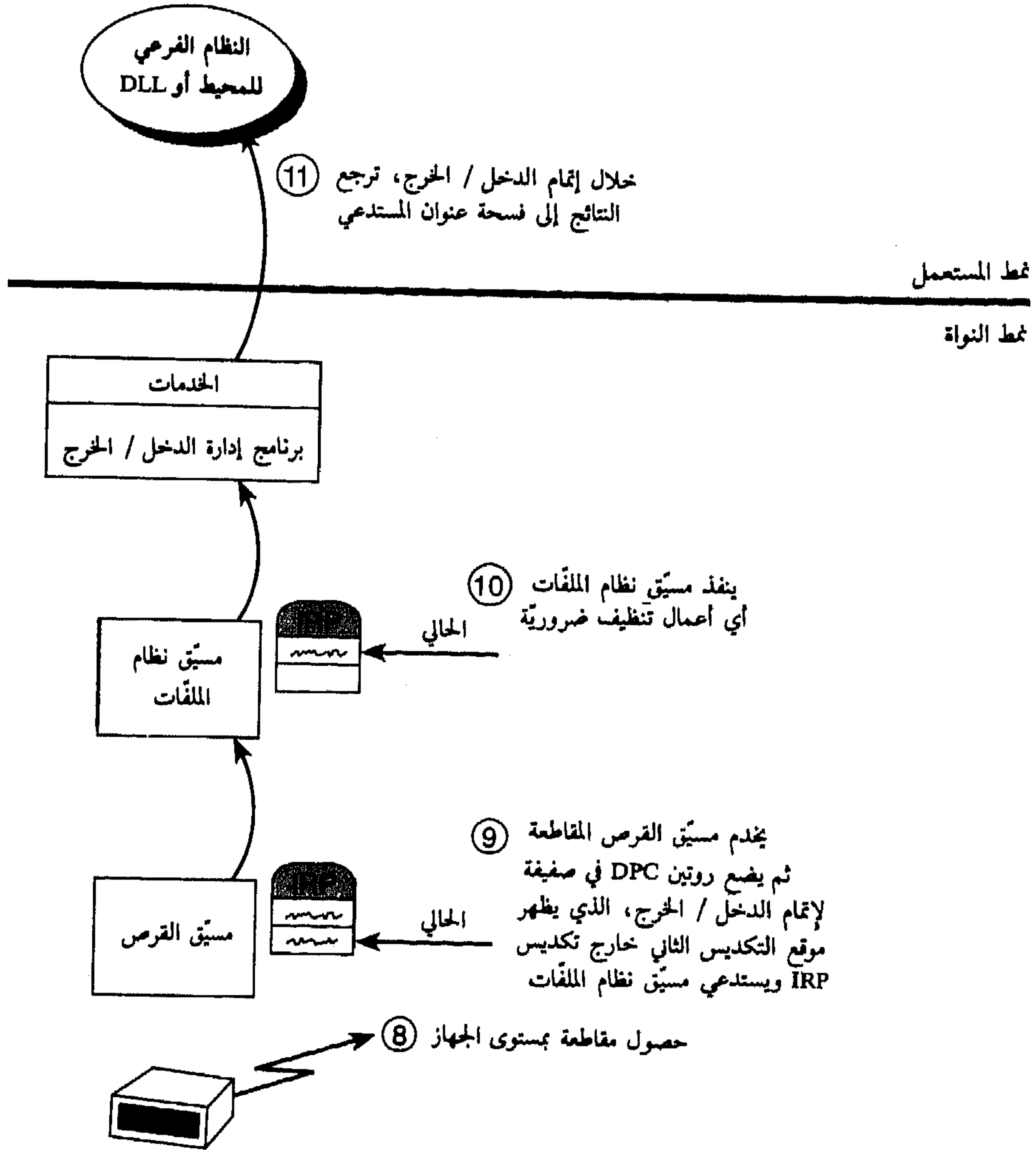
الشكل (8-16) إتمام طلب دخل / خرج مرتب في طبقات
