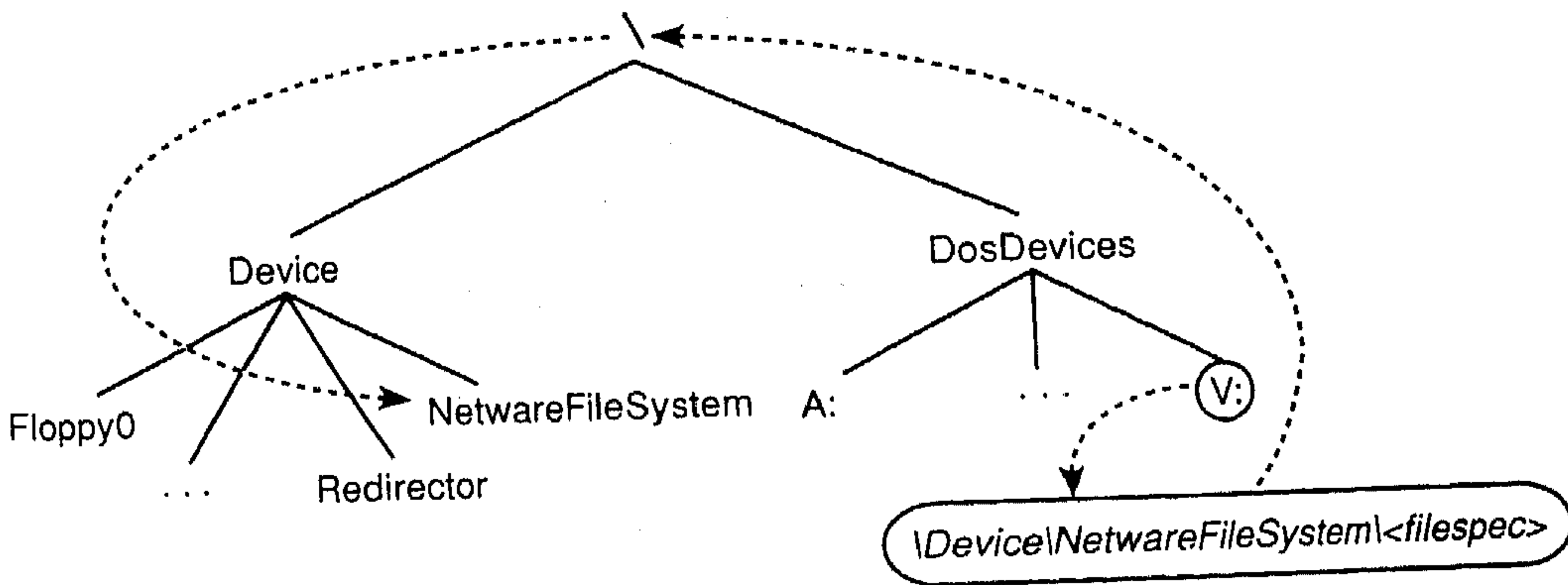
الشكل (10-9) التدقيق في إسم مورد شبكة
