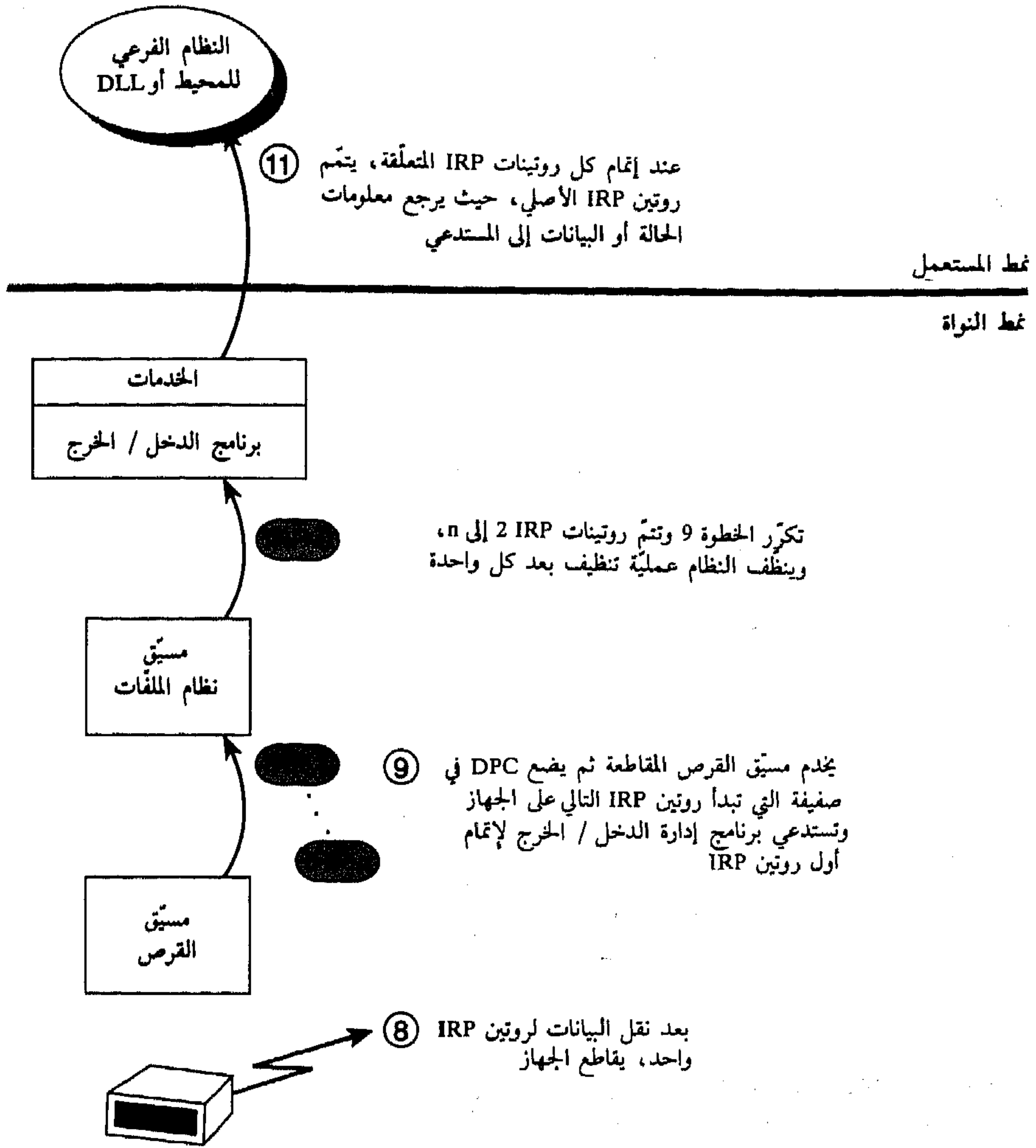
الشكل (8-18) إتمام روتينات IRP المتصلة
