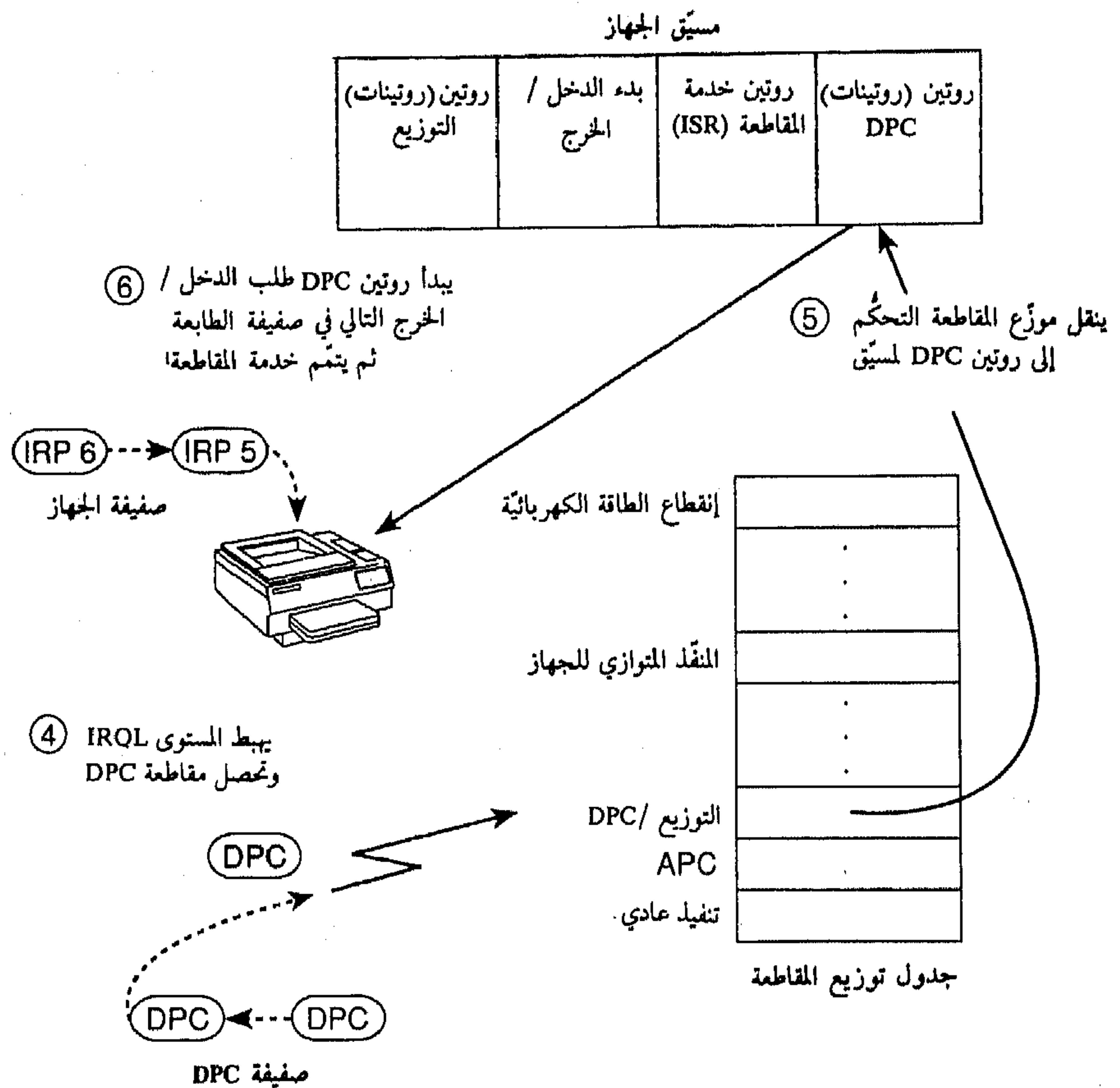
الشكل (12-8) خدمة مقاطعة جهاز (المرحلة 2)
