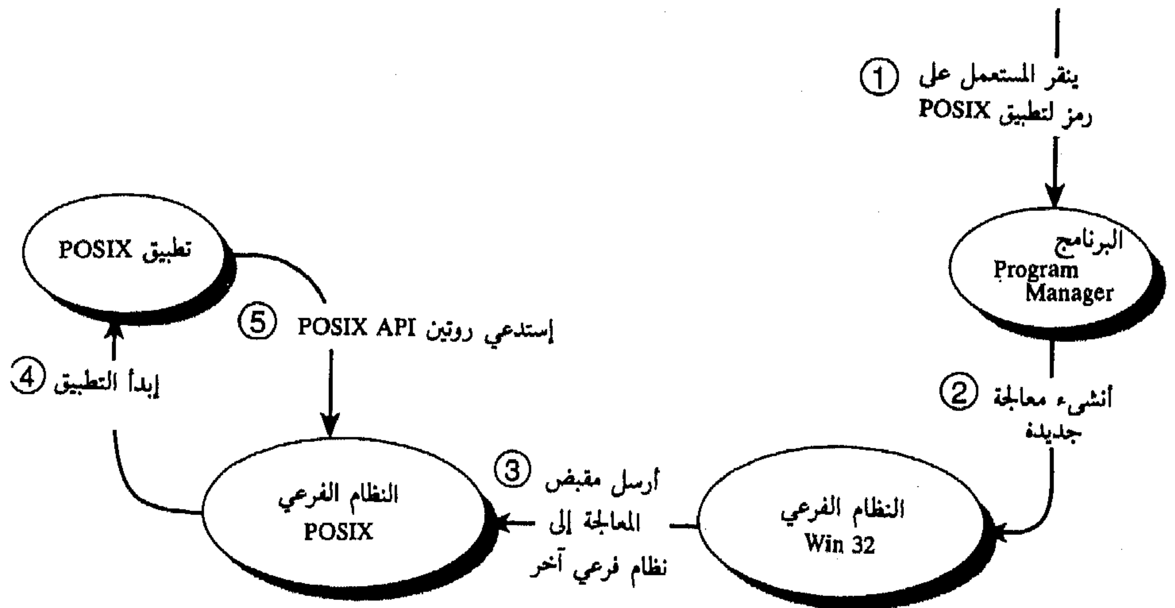
الشكل (5-12) بدء تطبيق غير Windows
