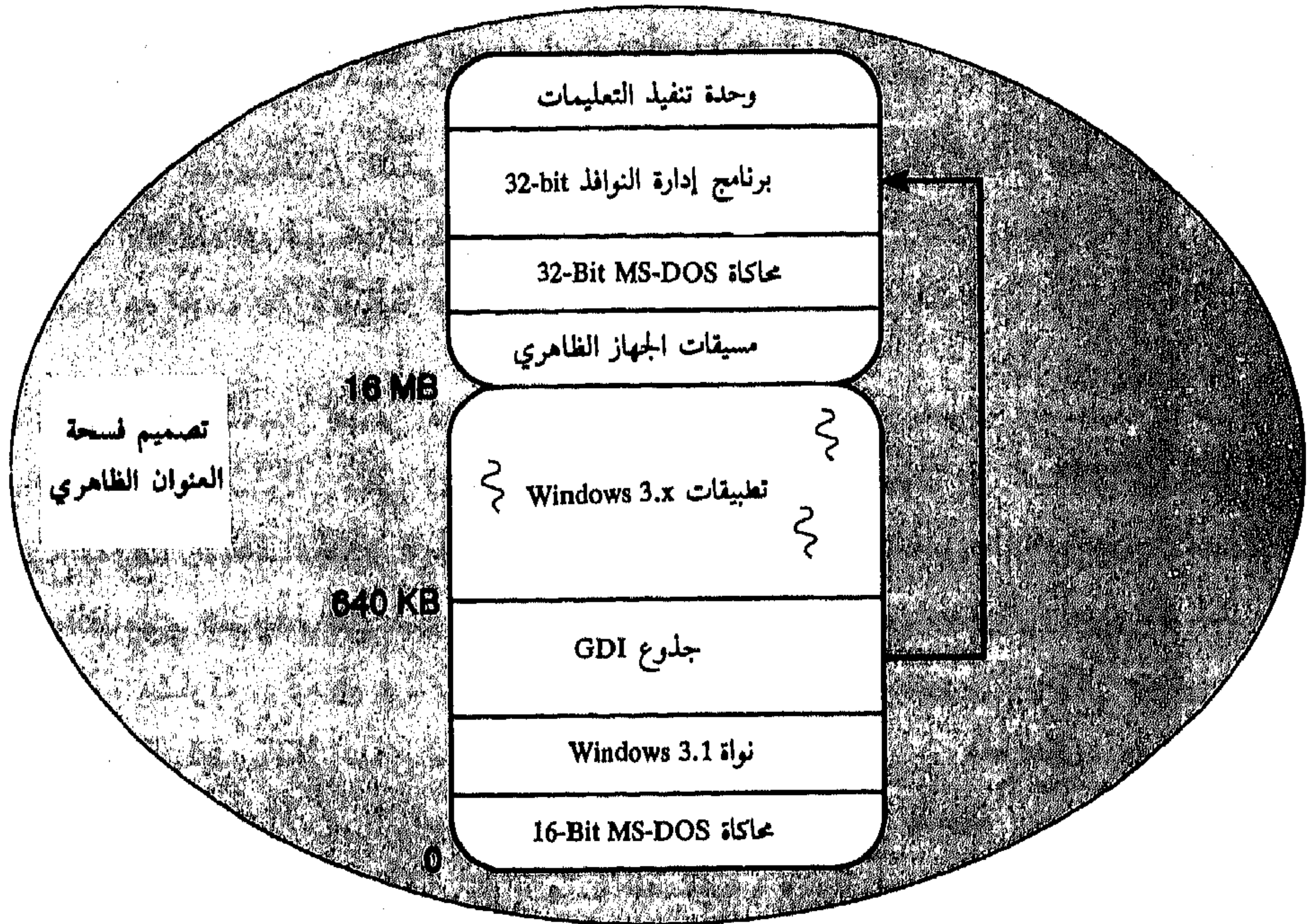
الشكل (19-5) 16-Bit Windows على Win 32 (WOW)
