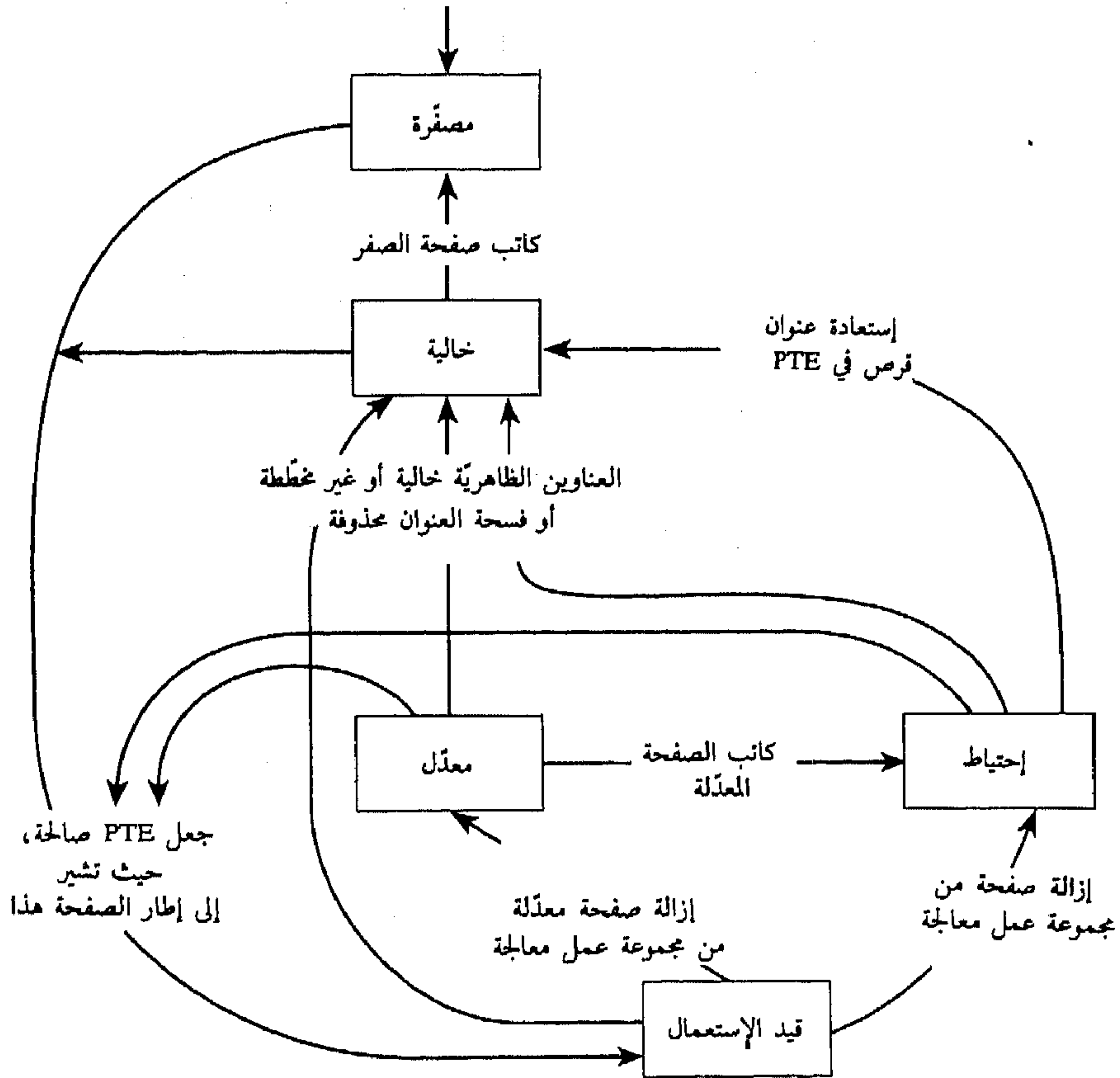
الشكل (15-6) مخطط حالة أطر الصفحة
