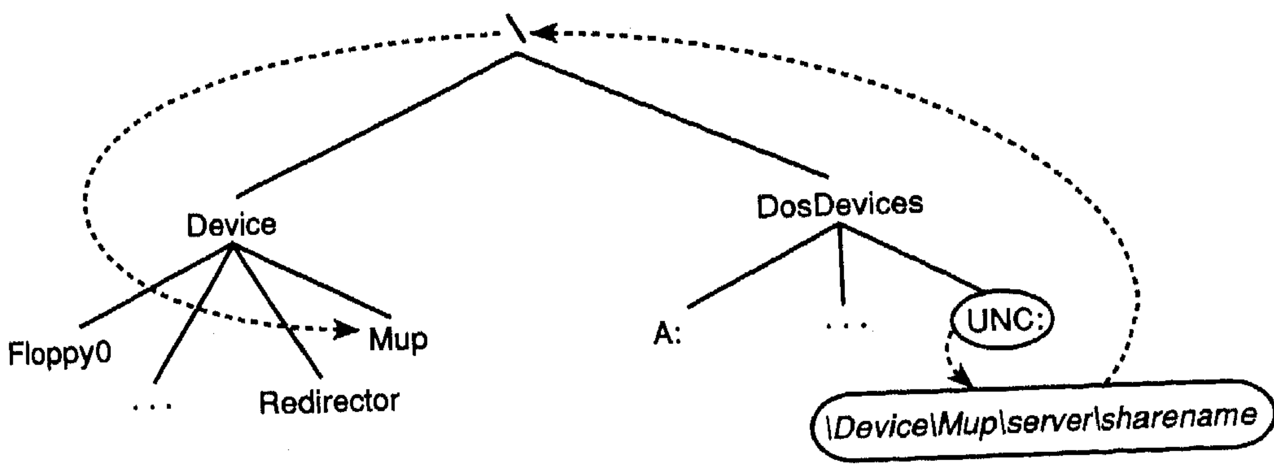
الشكل (12-9) التدقيق في اسم UNC
