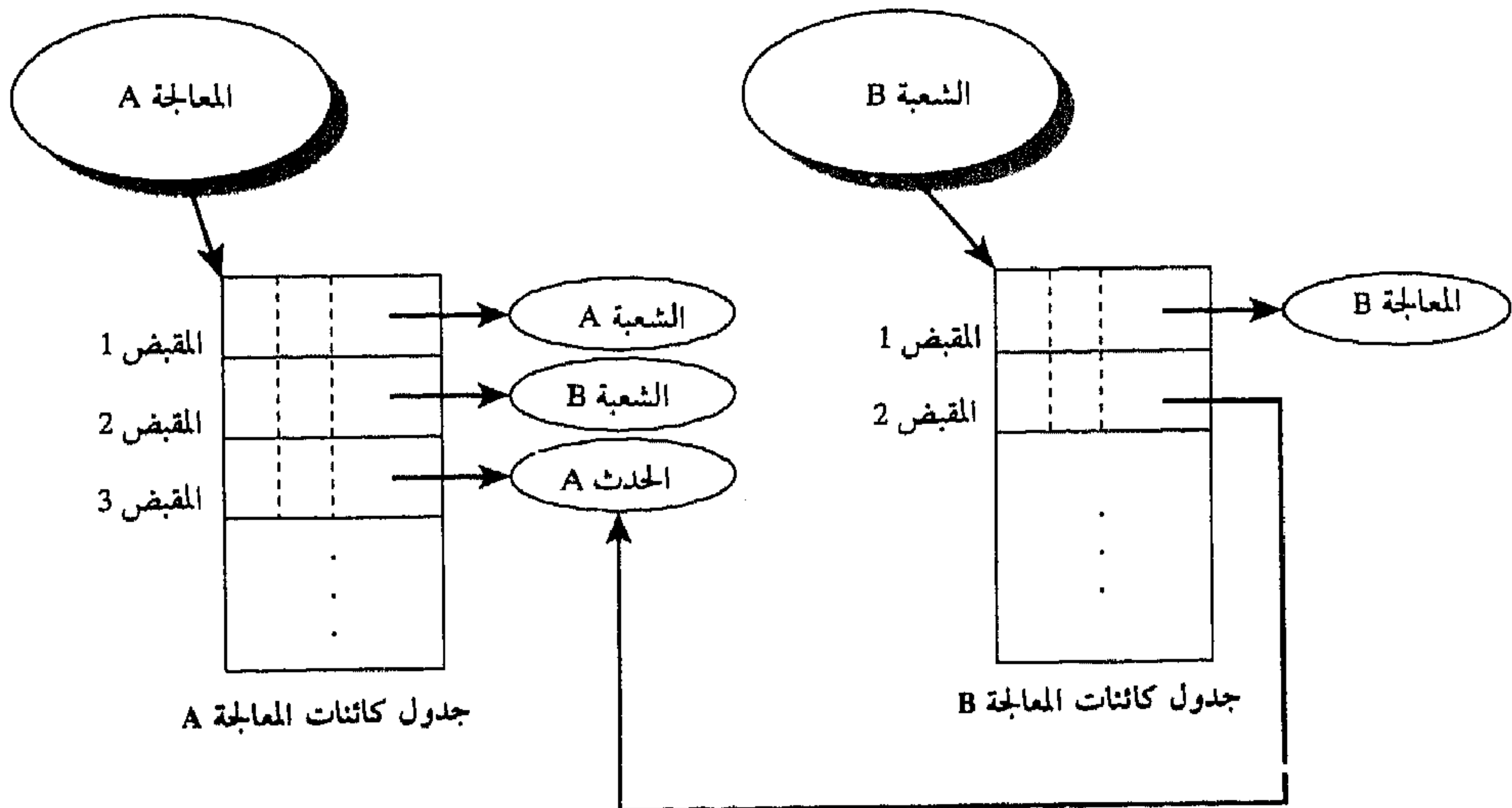
الشكل (7-3) مشاركة كائن
