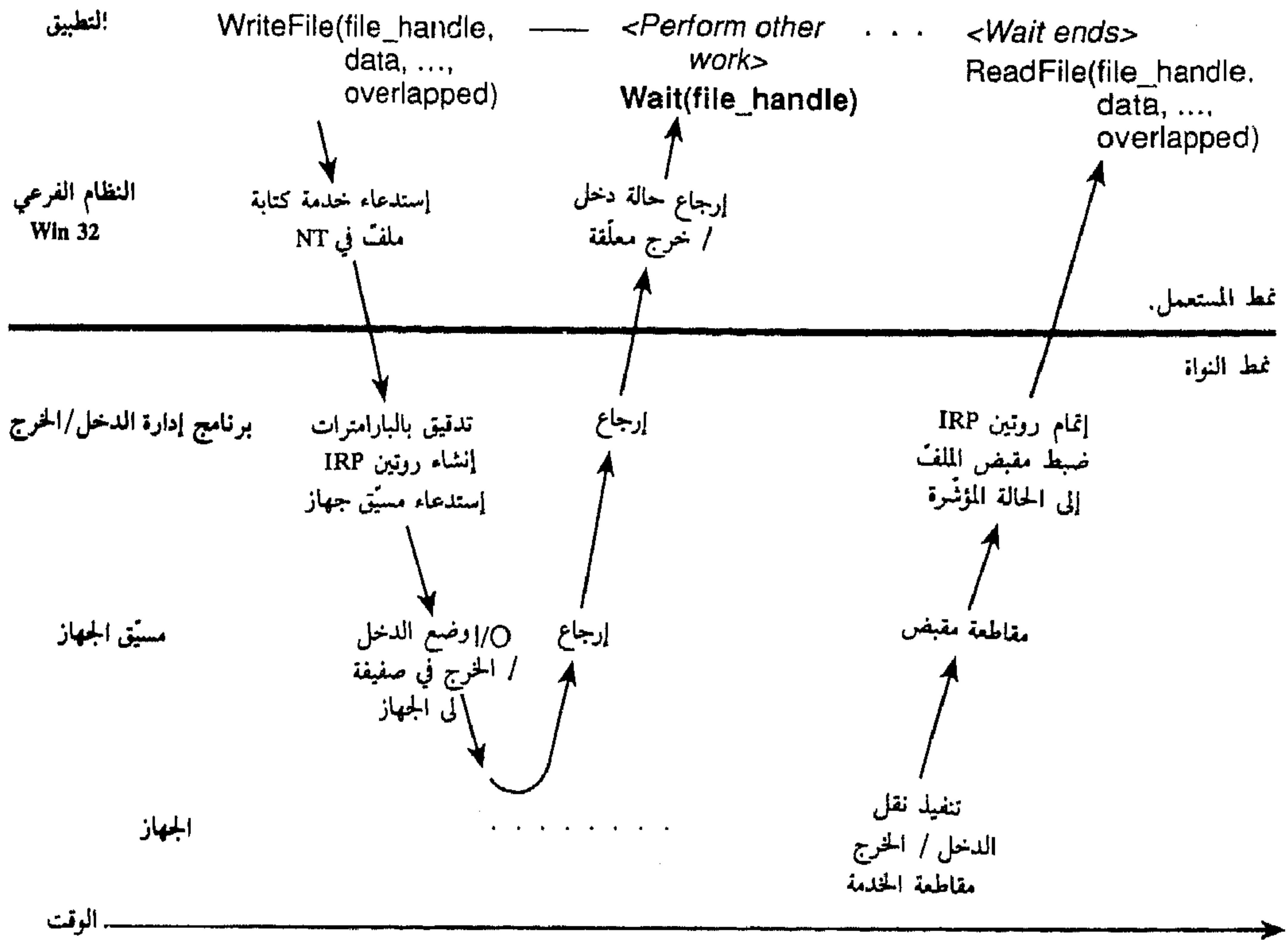
الشكل (6-8) الدخل / الخرج غير المتزامن
