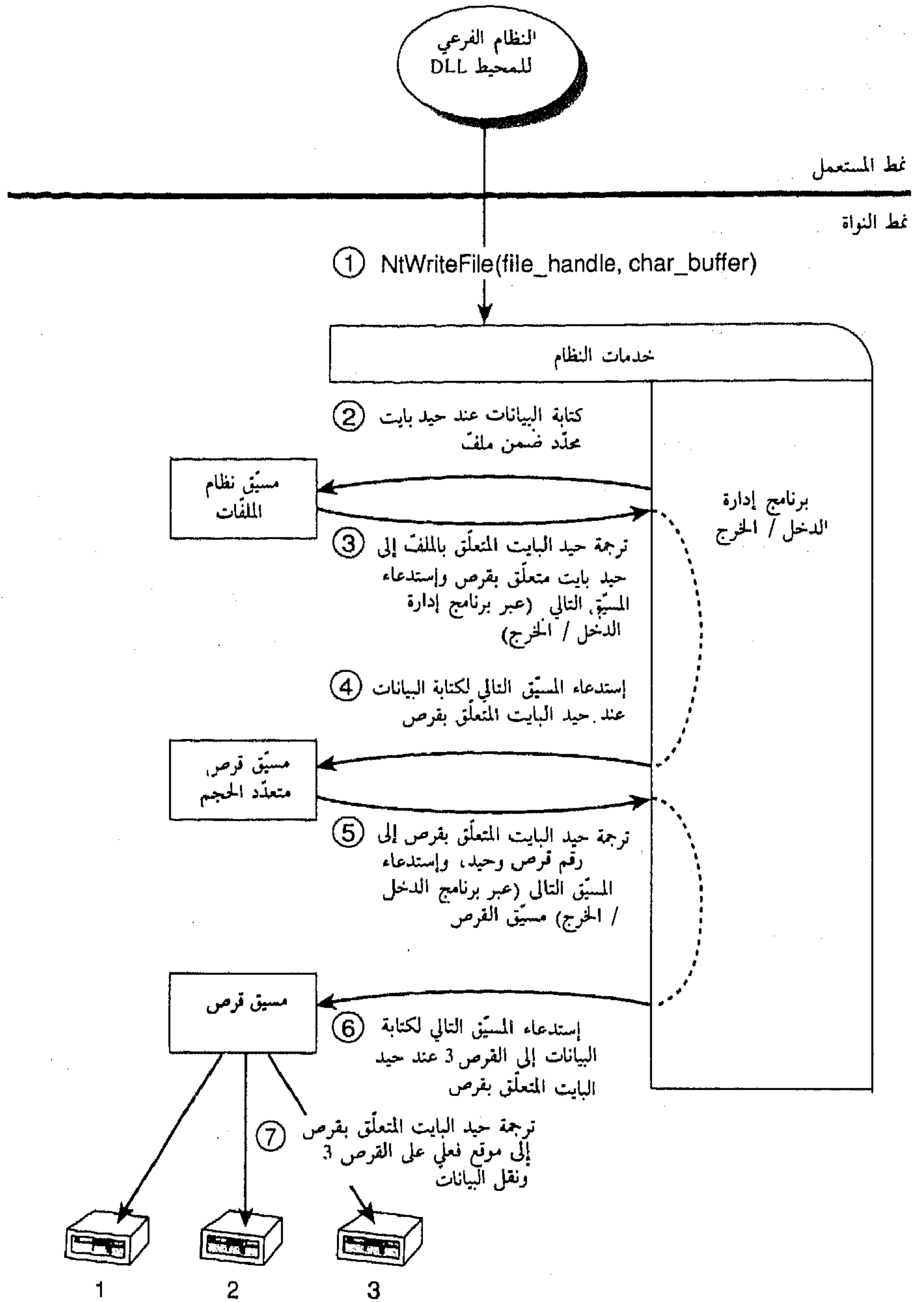
الشكل (8-23) إضافة مسيّق مرتّب في طبقات
