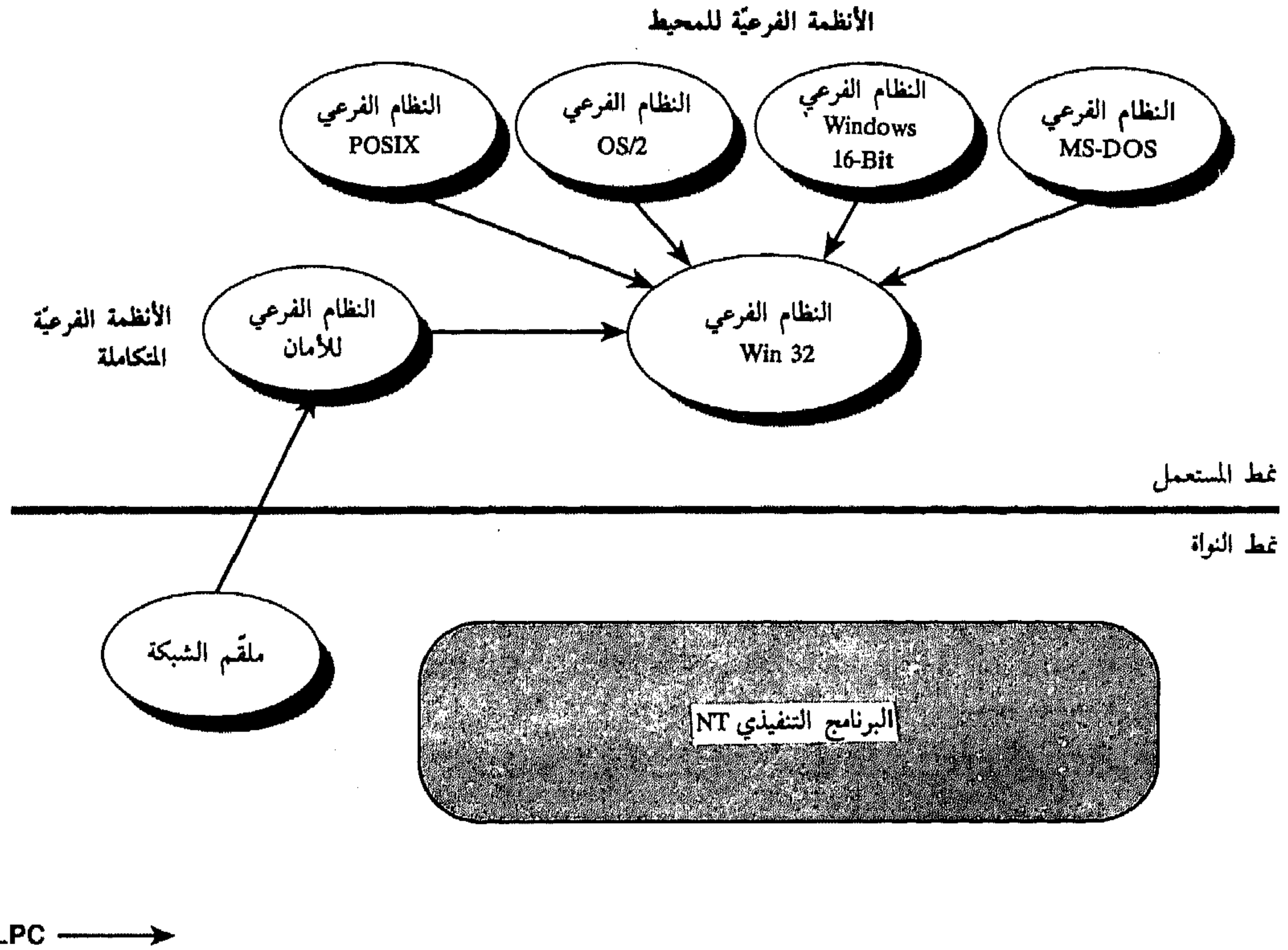
الشكل (1-5) الأنظمة الفرعية المحيية في Windows NT
