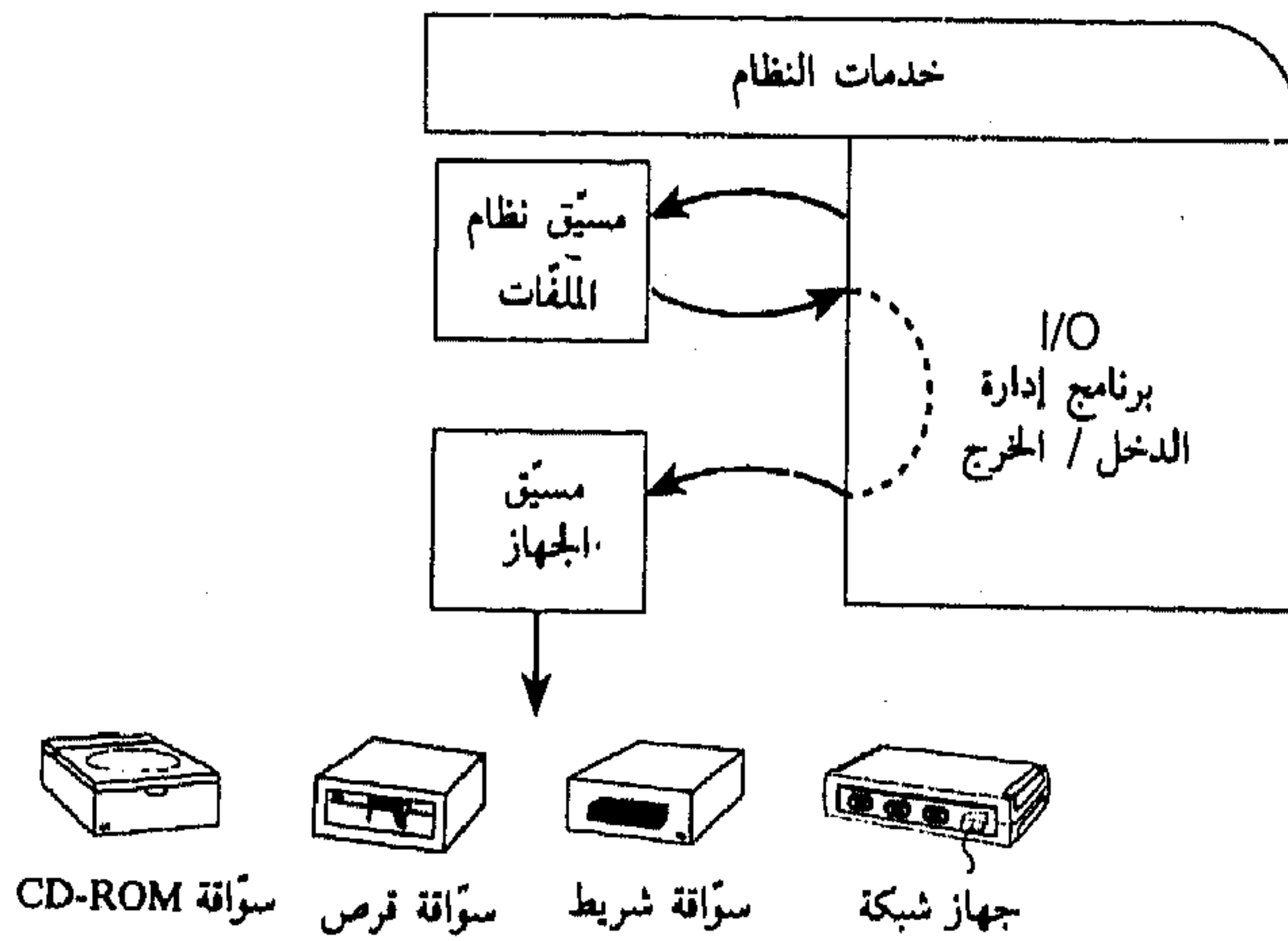
الشكل (4-8) دخول / خرج إلى ميق متعدد الطبقات
