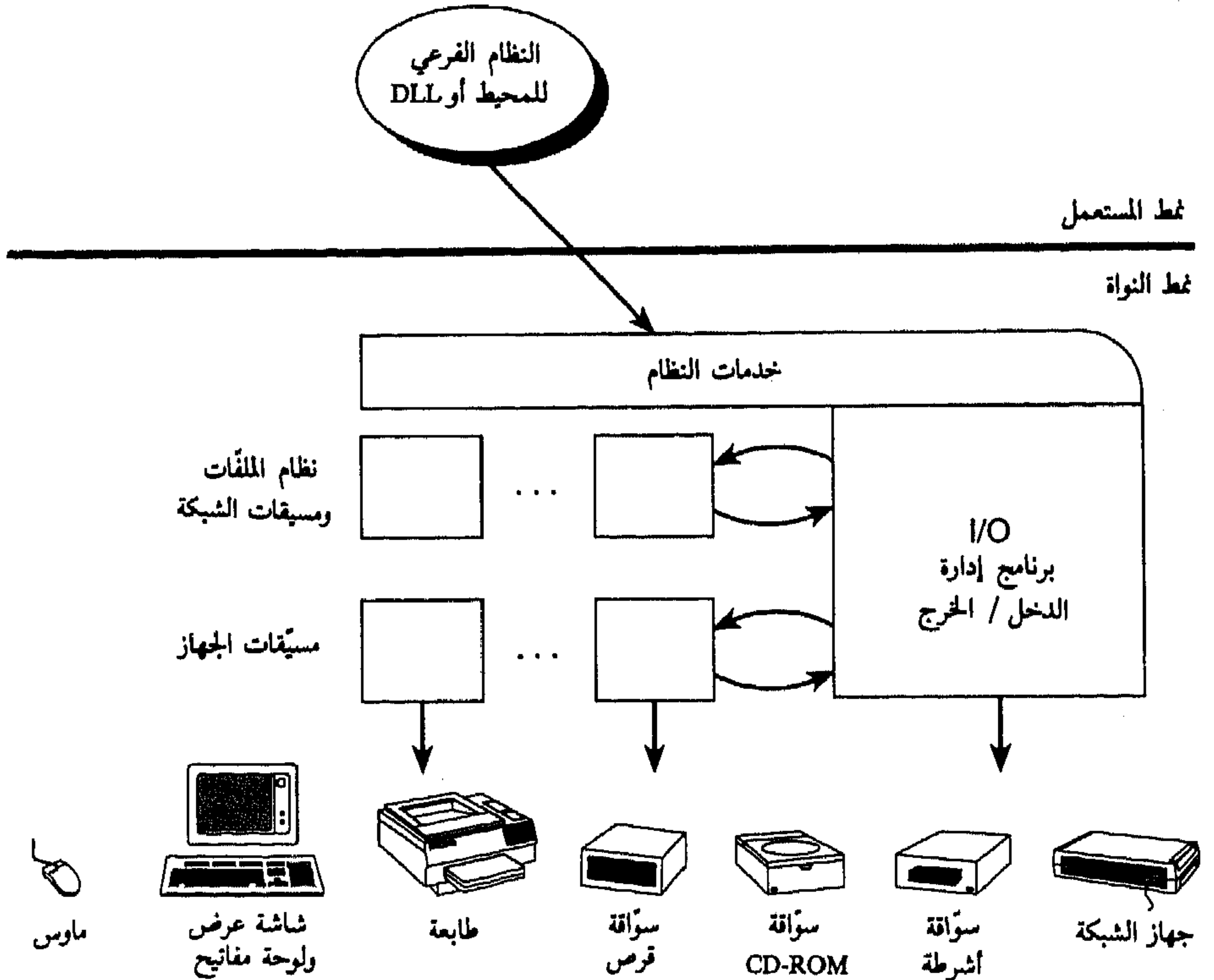
الشكل (1-8) أجزاء نظام الدخل / الخرج
