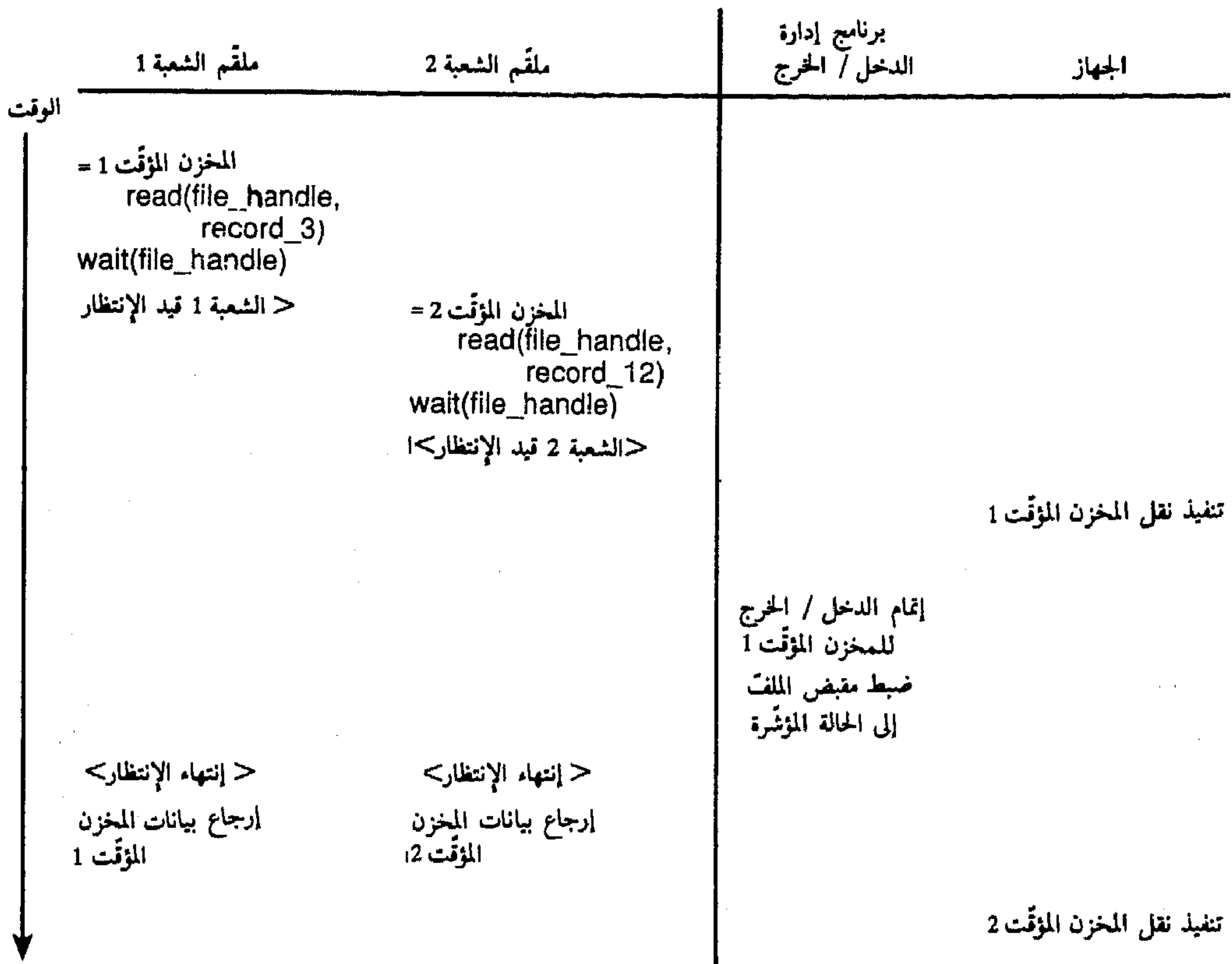
الشكل (19-8) الإستعمال الخطأ لمقبض ملف
