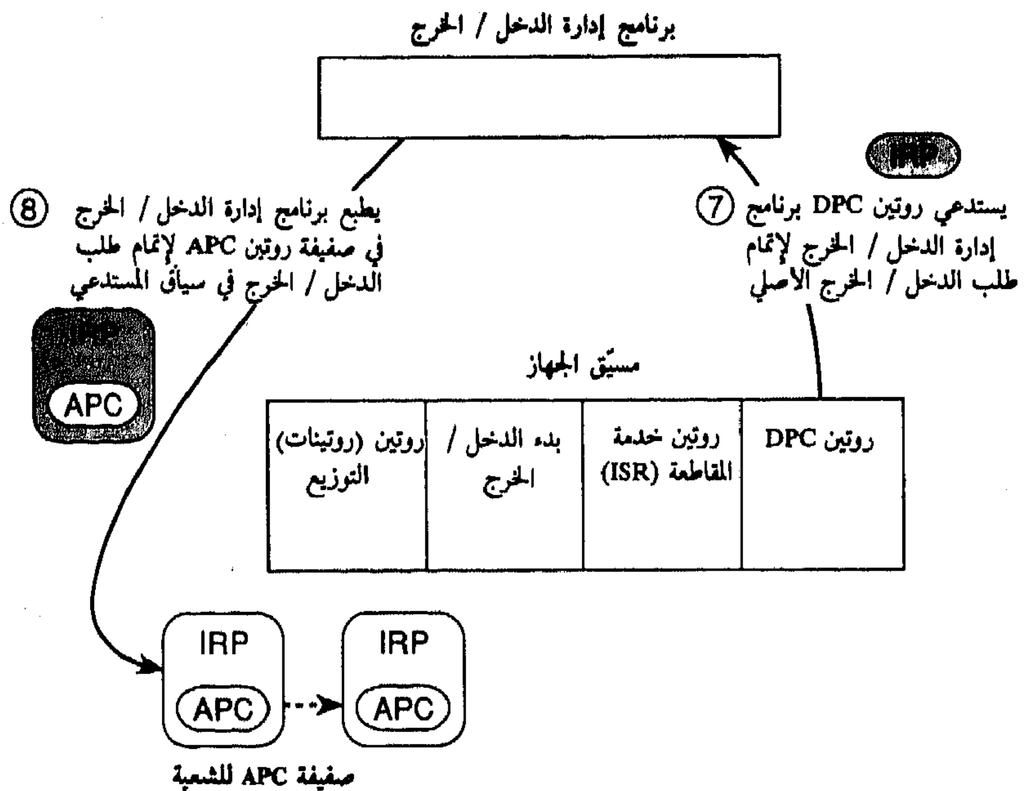
الشكل (13-8) إتمام طلب دخل / خرج (المرحلة الأولى)
