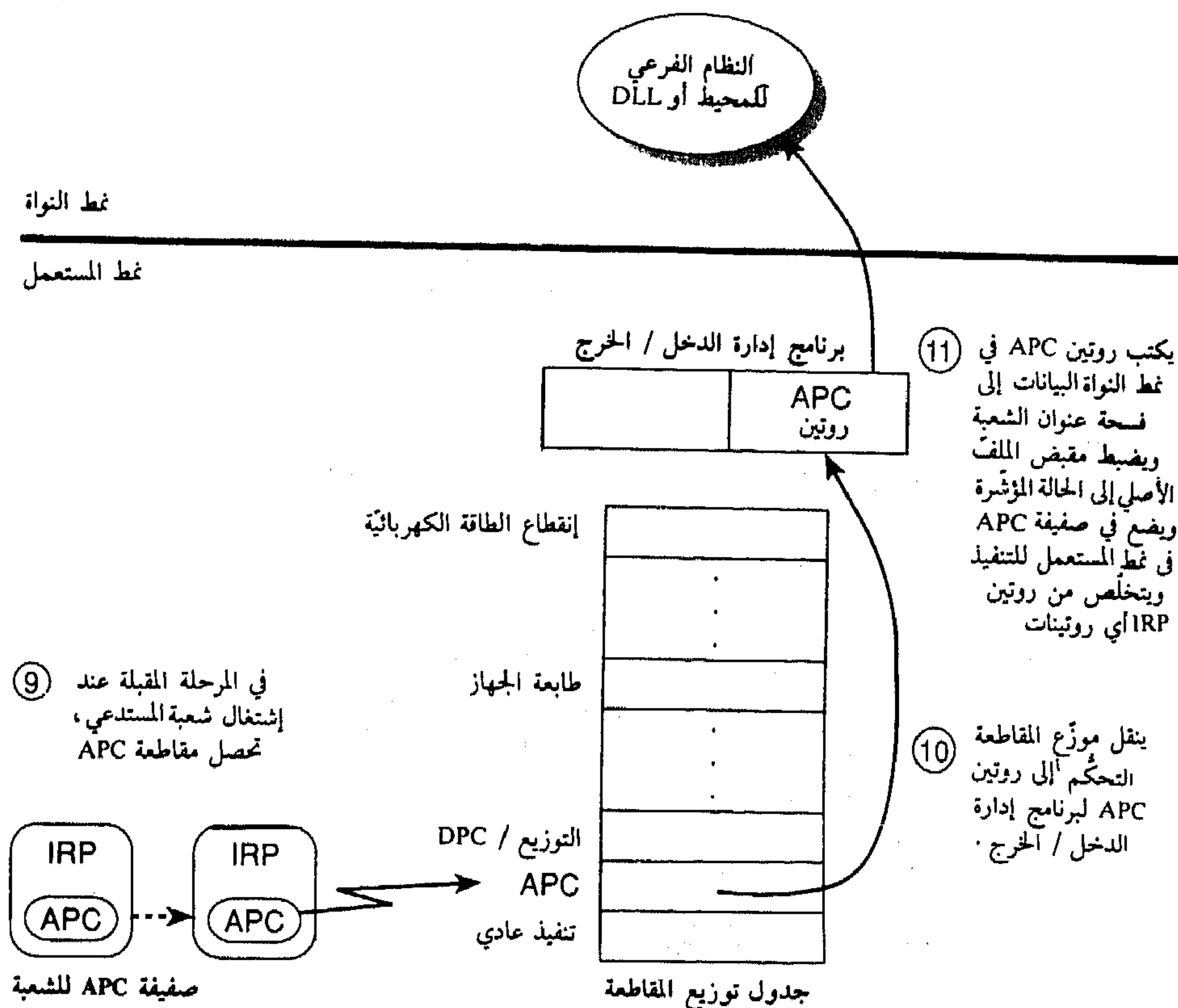
الشكل (8-14) إتمام طلب الدخل / الخرج (المرحلة الثانية)
