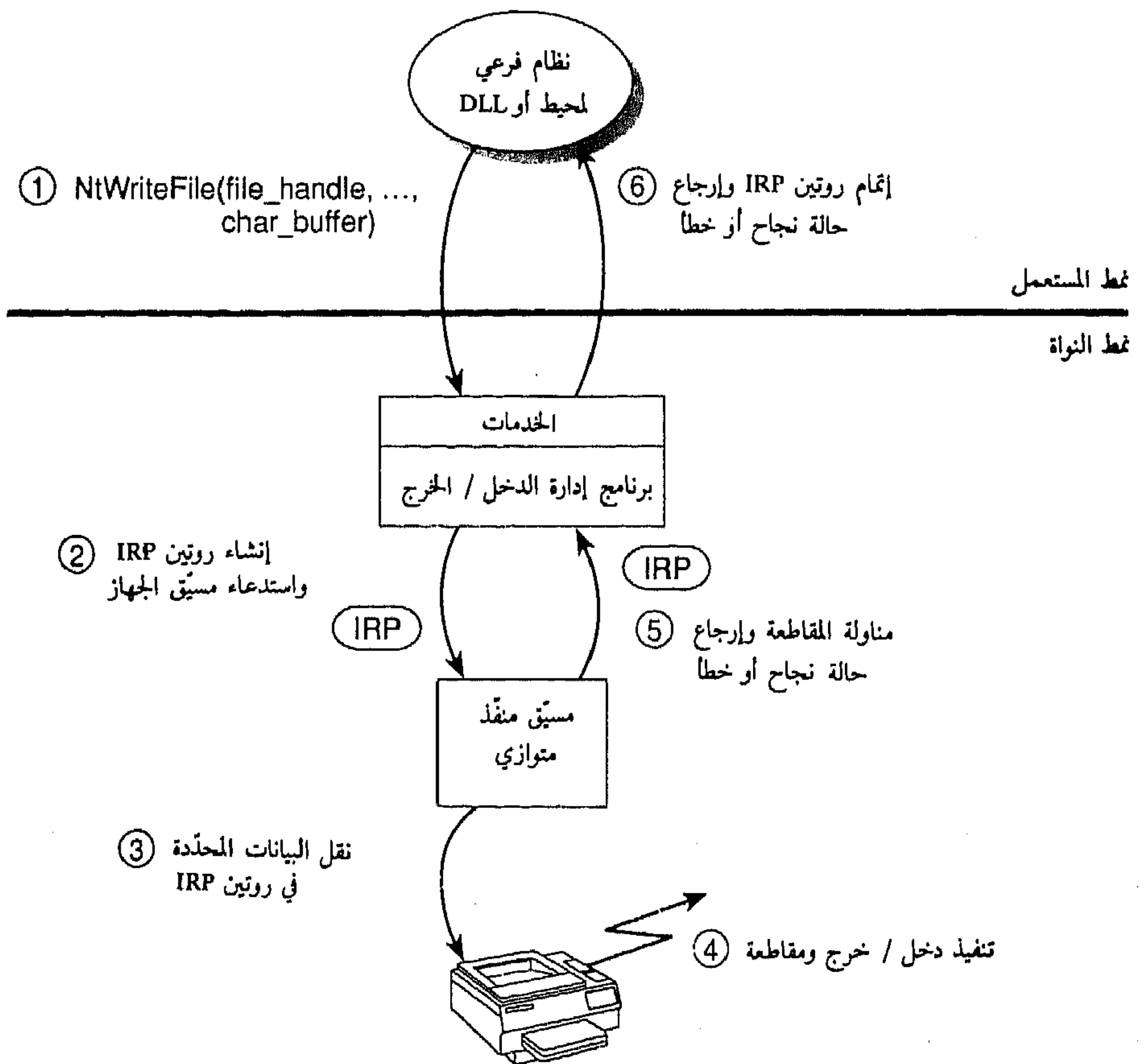
الشكل (9-8) وضع طلب متزامن في صفيحة وإتمامه
