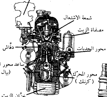
الكربوراتور أو العبايق أو محول التبخير
