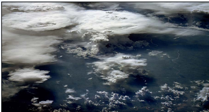
一张积雨云照片，取自于美国航空航天局。它就好像是被一只无形的手推进着
