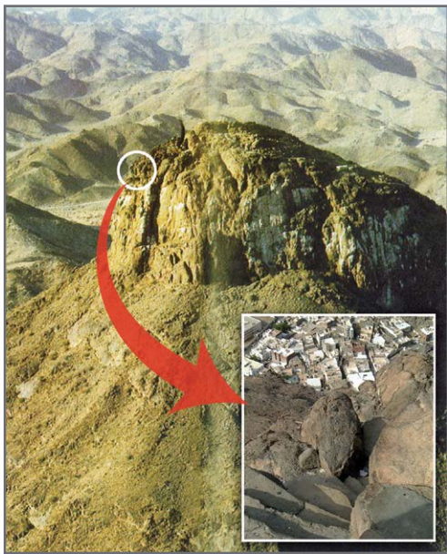
希拉山洞，位于麦加以东，距禁寺4公里的“努尔”山上，海拔约为634米
