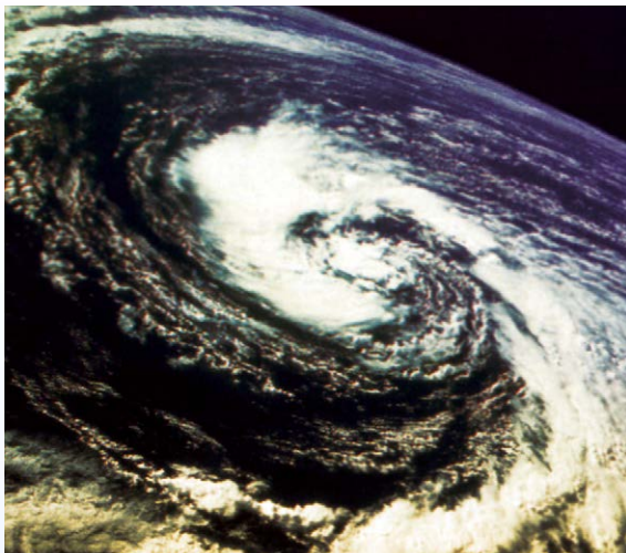
大气层的图像，包围着它的是云和风
