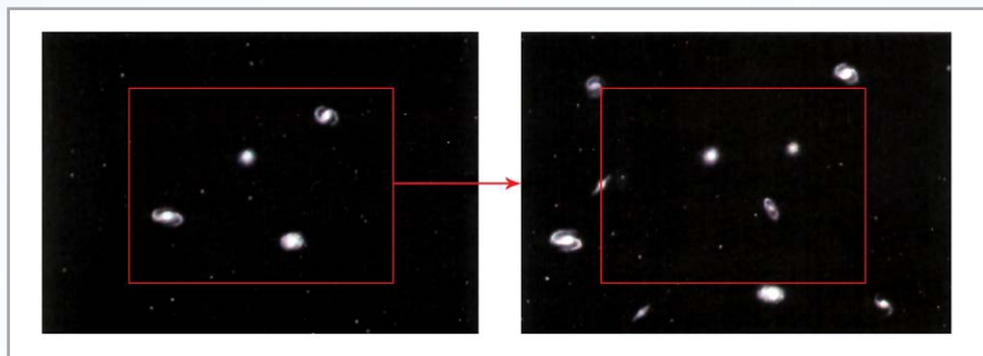
这张照片显示的是，星系与星系团之间的距离在不断增加，由此证明宇宙正在膨胀之中
