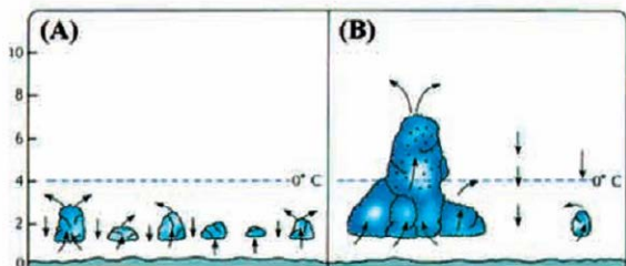
图 (A) 表示小云片，即积云。图 (B) 许多积云汇聚在一起，形成的大云团的向上引力增大。于是云体向上聚集。
