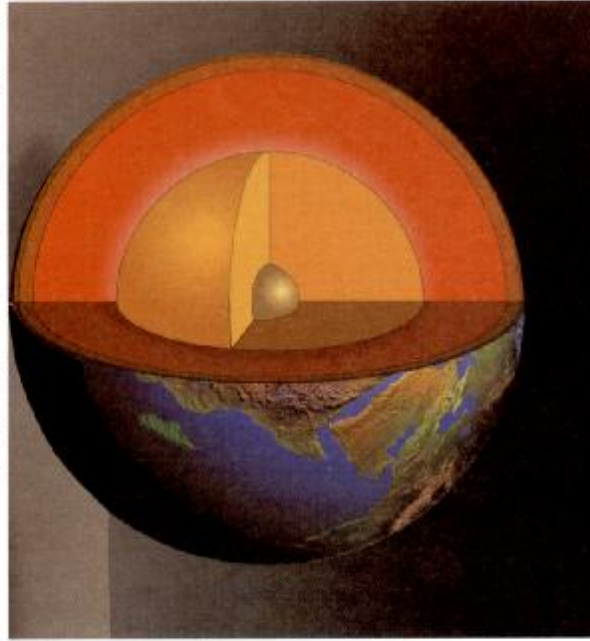
● الحديد المنصهر في لب الأرض
