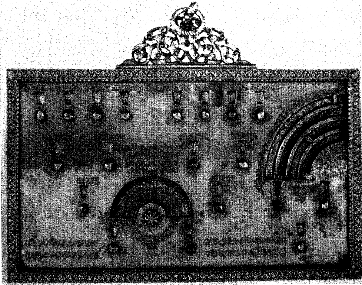
الصورة ١٨-٨ آلة هندسية من سوريا أو من بلاد ما بين النهرين مصنوعة من النحاس الأصفر والأحمر، مطعمة بالفضة والذهب، بتوقيع <محمد بن خُتْلُج الموصلي> بتاريخ ٦٩٣ هـ / ١٢٤١ م. [بترخيص من المتحف البريطاني - لندن].
