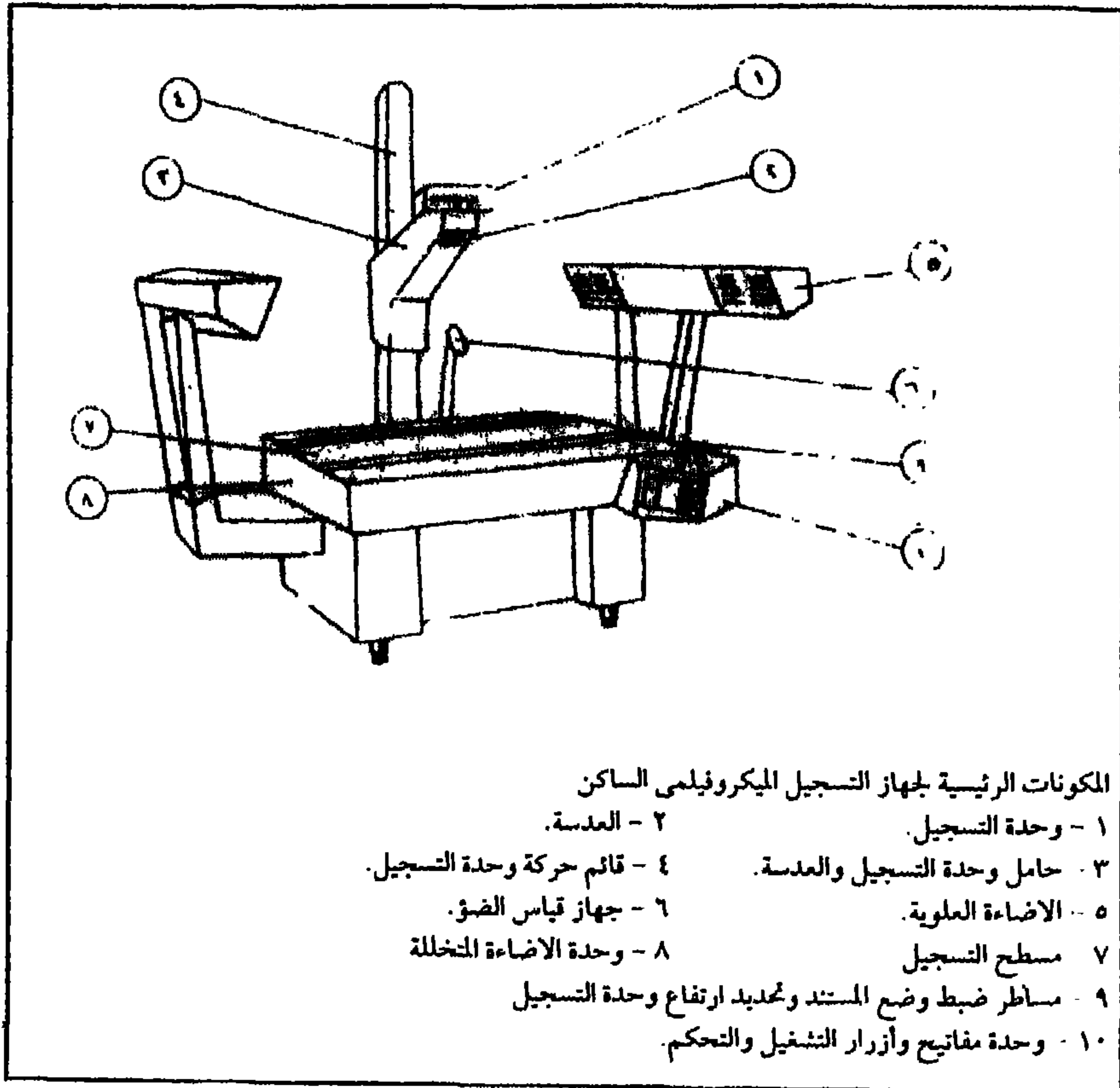
شكل (٦٣) أحد أنواع أجهزة التصوير الميكروفيلى
