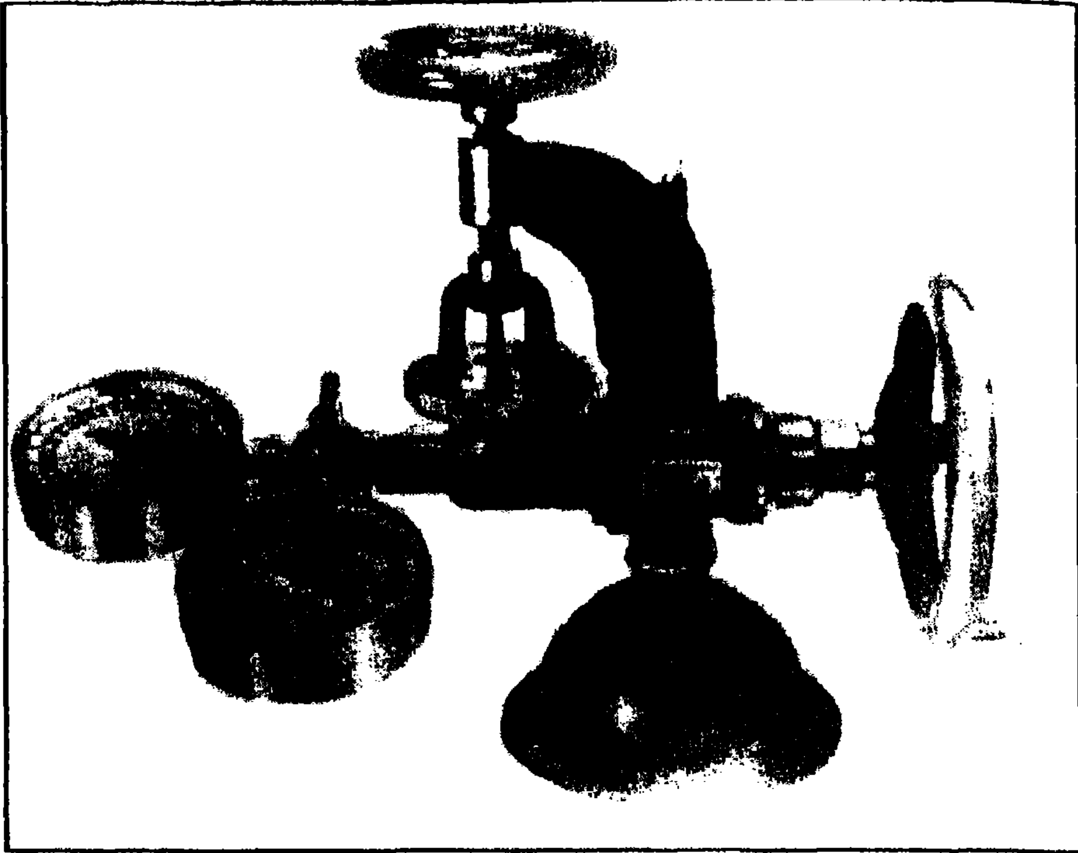
شكل (٢٨) جهاز Mullen لقياس قوة الانفجار
