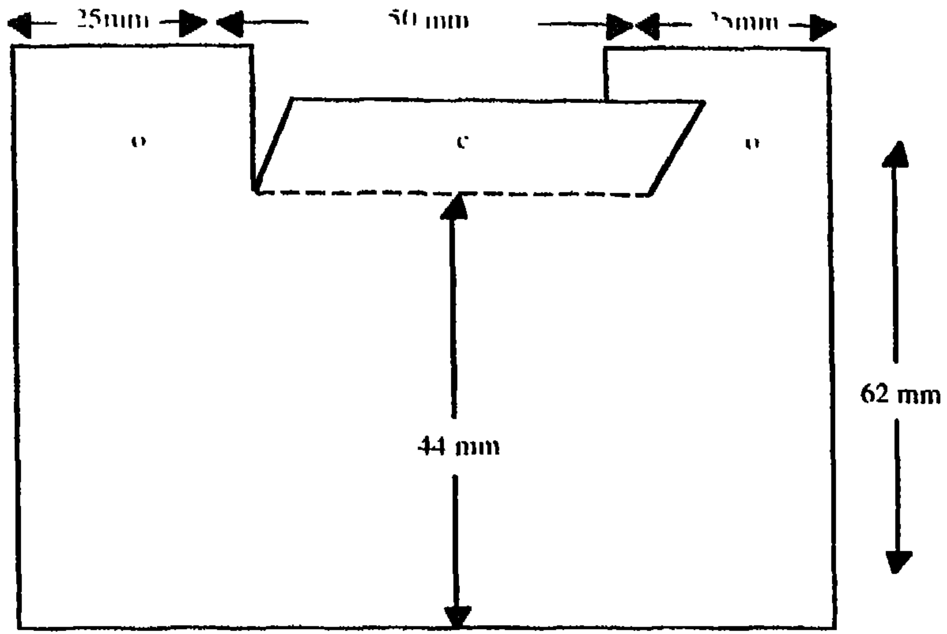
أبعاد عينة الورقة المستخدمة شكل (٢٧) يوضح كيفية تقدير قوة التمزق للورق
