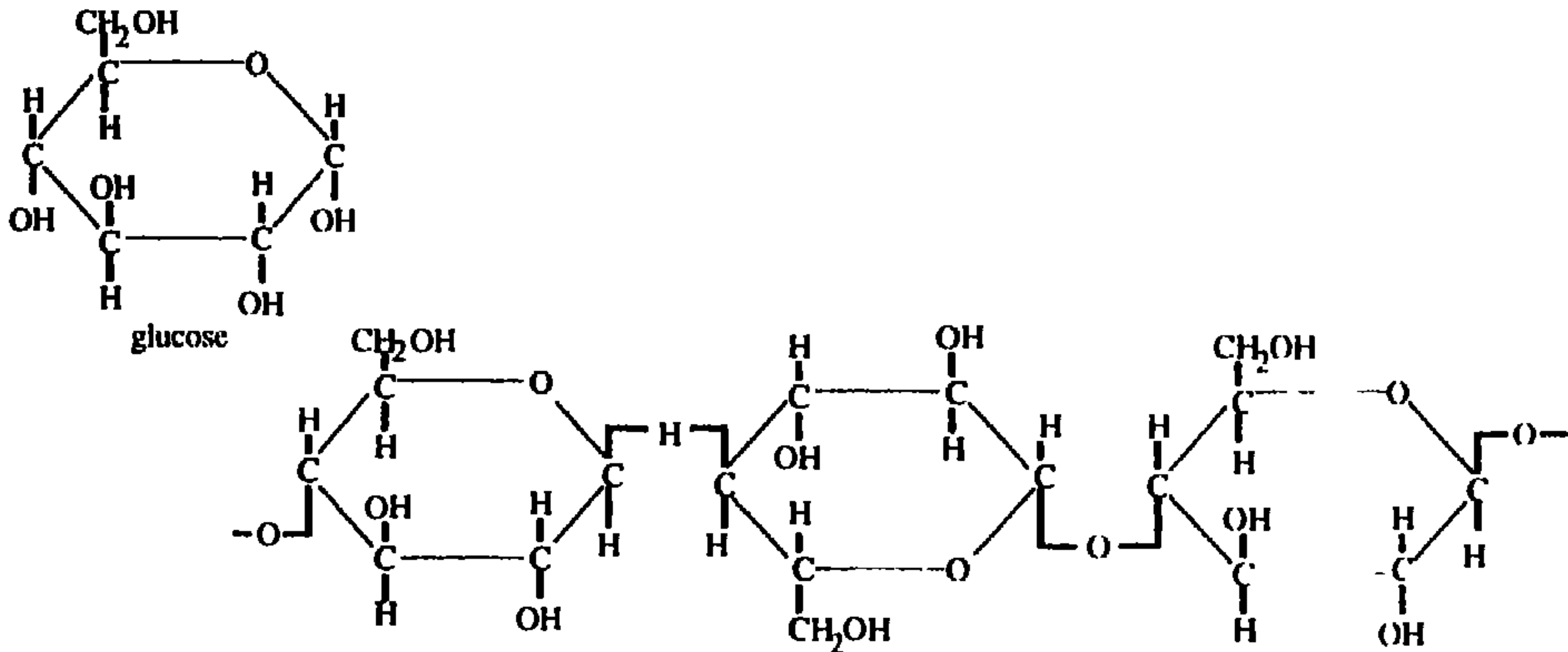
شكل (١) تتابع الوحدات في ليفة السليولوز «Structur of Gllubse fibre»
