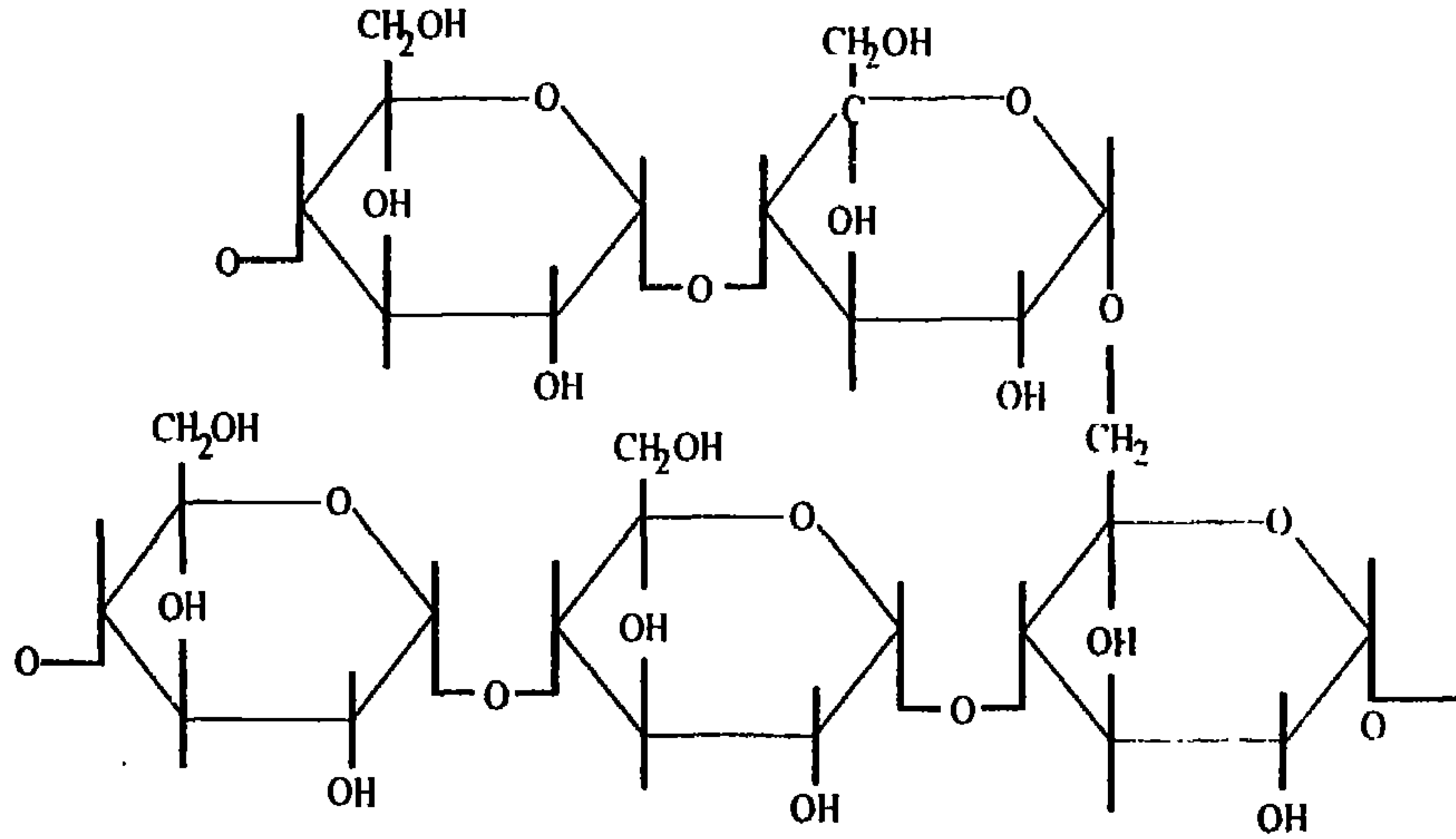
السلسلة المتفرعة في تركيب الاميلوبكتين
