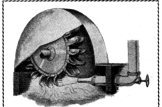
عجلة مائية يديرها ماء خارج بانفداع شديد من فوهة . والعجلة والماء مغلقتان في علبه . وتسمى هذه العجلة بعجلة بلتن Pelton وهي مبتدعها . وهي تنفع لمساقط الماء العالية التي مقدار مائها غير كبير .
