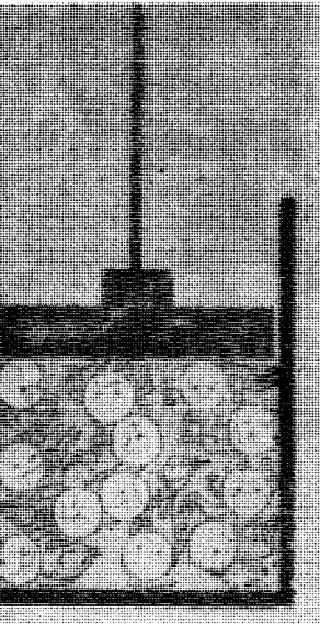
زحمتنا الجزيئات في حجم أصغر ، فزاد دقها جدران الوعاء ، فزاد الضغط .
