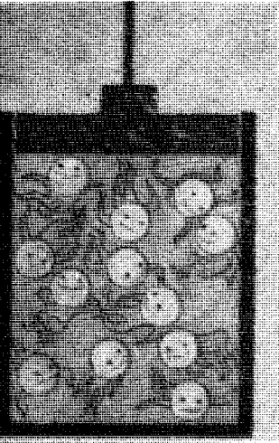
جزيئات من الغاز ، في حركة دائسة .
