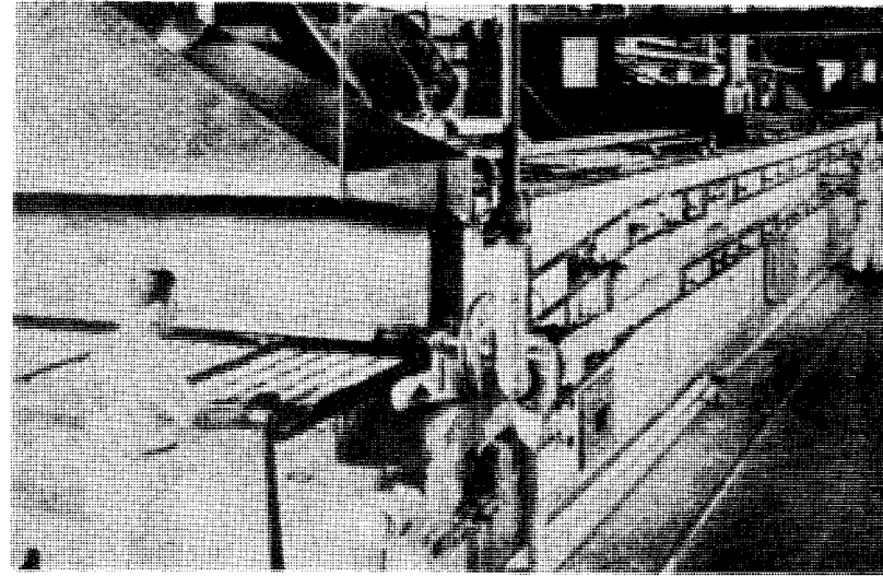
الفرن ، وهو طويل ، وقد بلغ طوله ٣٠ قدما أو يزيد ، وفيه تسير الصواني بالأرغفة من طرف الى طرف ، فلا تصل الى الطرف الآخر حتى تكون قد تم نضجها .
