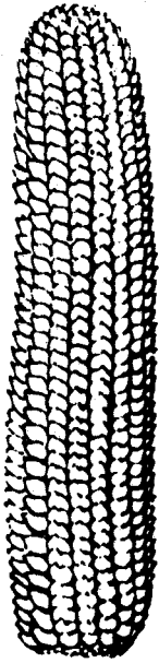
ذرة النشا
