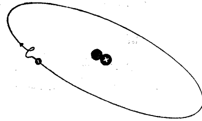
ذرة ادرجين ثقيل : نواة ( بروتون ونيوترون ) يدور حولها الكترون
